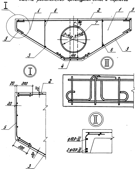
Схема расположения арматурных сеток и каркасов
