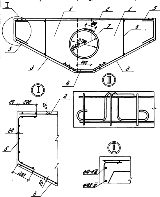
Схема расположения арматурных сеток и каркасов
