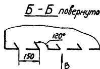
Рис. 1 Водуохраспределитель перфорированный круельный тип ВЛК1.
