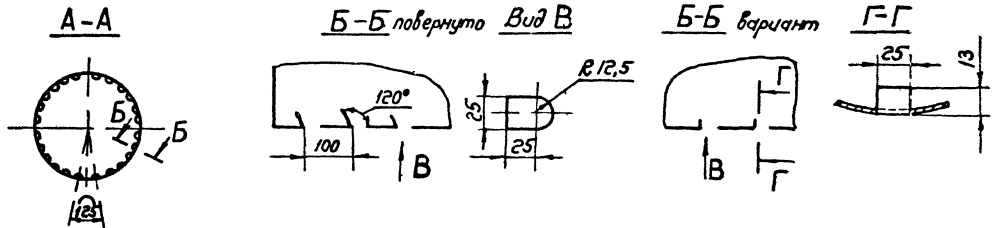
Рис 3. Воздухораспределитель перфорированный круглый тип ВЛКЗ
