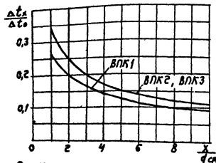
Рис 12 Максимальные относительные избыточные температуры в струе
