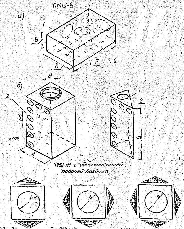
ПМШ-Н2 с двухсторонней подачей воздуха ПМШ-Н3 с трехсторонней подачей воздуха ПМШ-Н4 с четырехсторонней подачей воздуха
