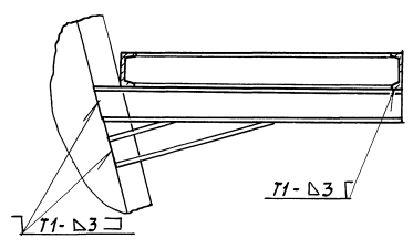
Д-Д (1:10)
