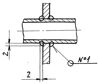
Д-Д (1:1) ○
