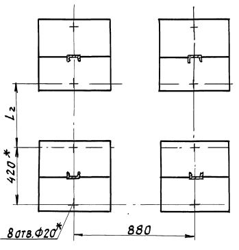
Б-Б (1:15) (1)
