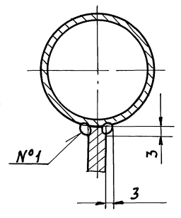
Г-Г (1:1) ○
