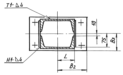
Б-Б
