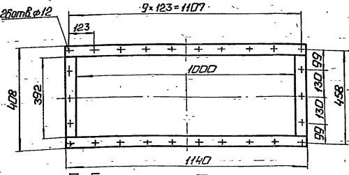
Вид А 9 × 123 = 1107
