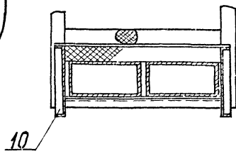
Вид Ж лист 1 М1:1
