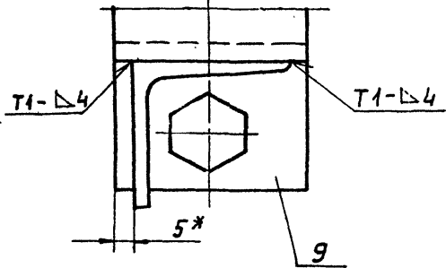
Вид Ж М 1:1
