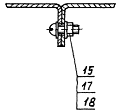
Б-Б лист 1 M 1:1
