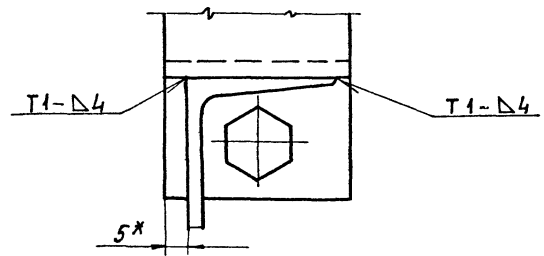
Вид Ж лист 1 М1:1
