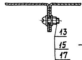
В-В лист 1 M1:2
