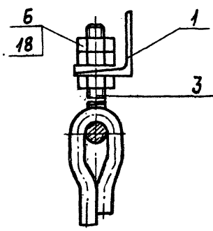
Вид Д М 1:2
