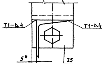
Вид Ж лист 2 М 1:2
