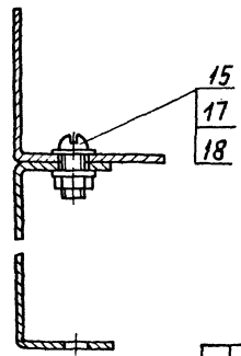
E-E M 1:1
