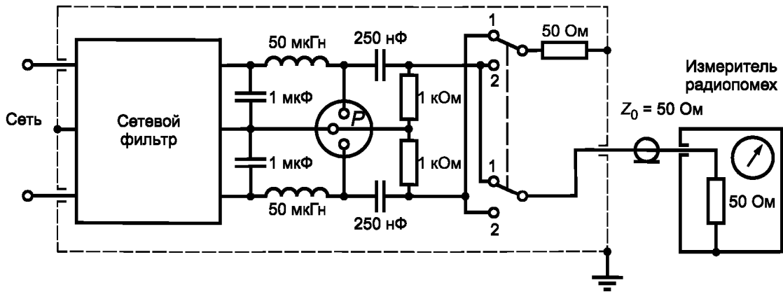
P — разъем для подключения испытываемого устройства
