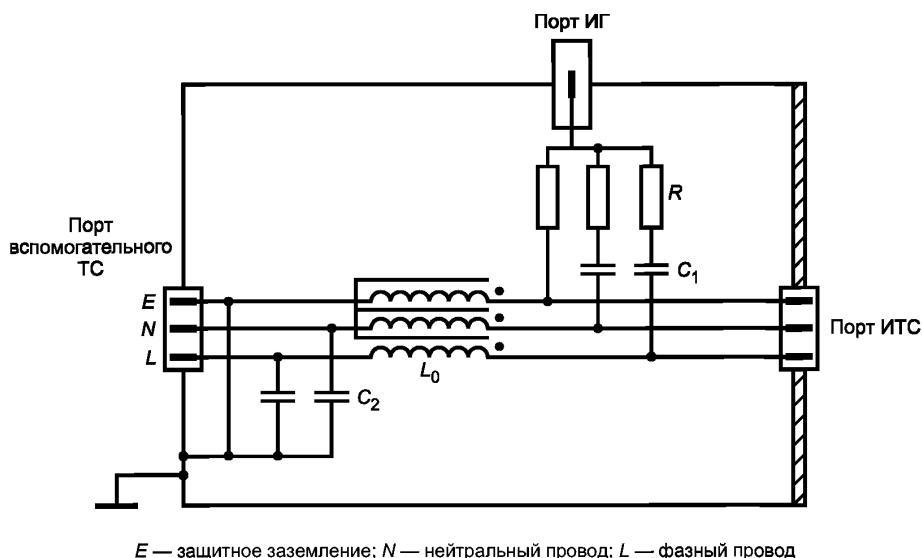
Рисунок 6 — Упрощенная схема устройств связи/развязки типов УСП-С1, УСП-С2, УСП-С3, применяемых при вводе помехи в неэкранированные кабели электропитания
