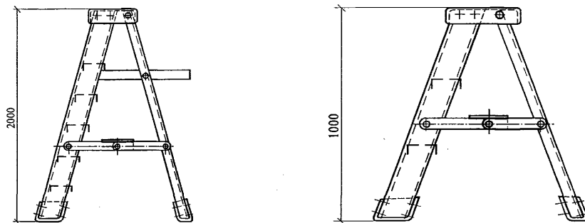
Рисунок 7 – Лестницы-стремянки
