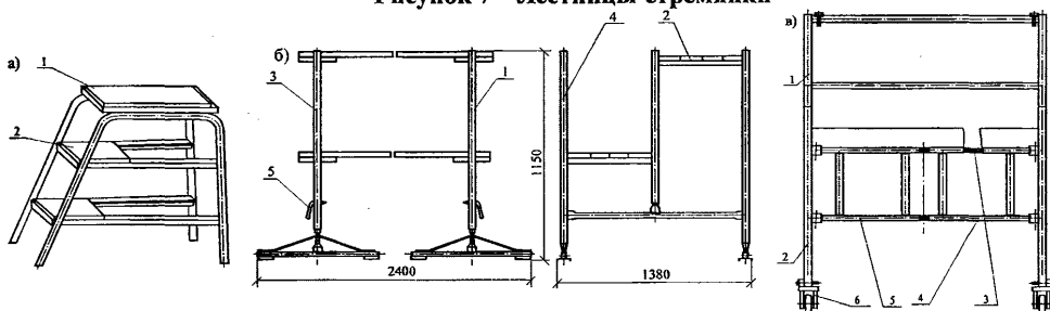
Рисунок 7 – Лестницы-стремянки
