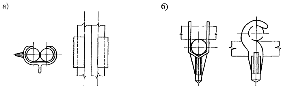
Рисунок 3 — Фиксаторы защитного слоя бетона для горизонтальной арматуры
