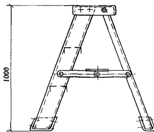
Рисунок 12 – Лестницы-стремянки
