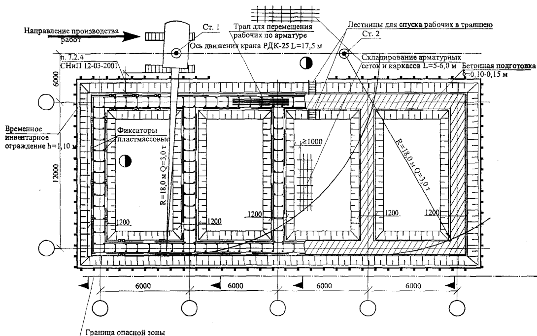
Рисунок 1 – Схема установки арматурных каркасов в ленточных фундаментах
