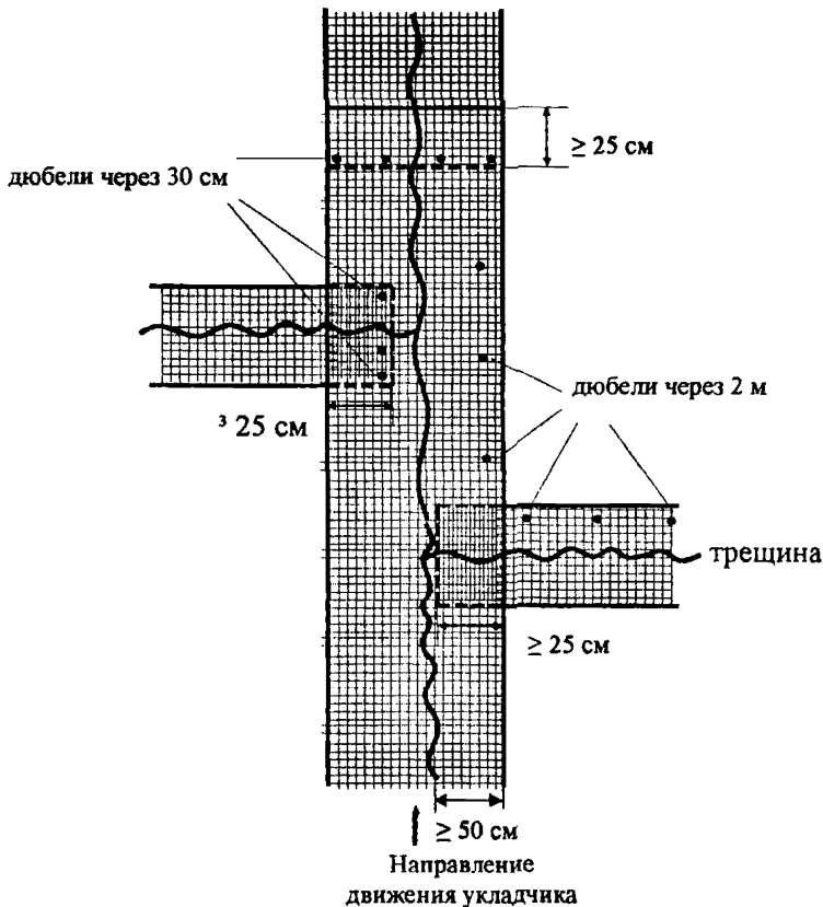
Рисунок 1 – Схема расположения полотен геосеток при локальном армировании
