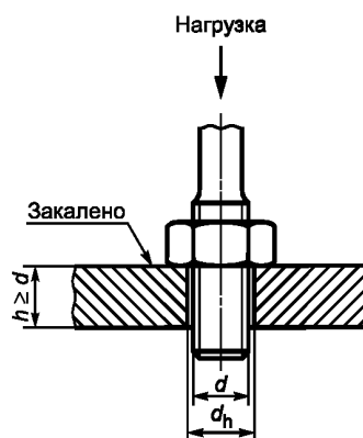
Рисунок 2 — Испытание на осевое сжатие
