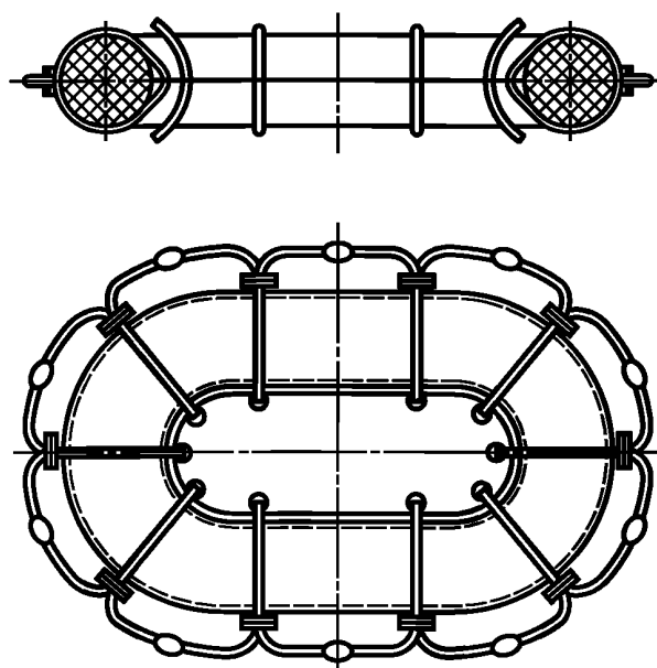
Рисунок 1 — Спасательный прибор
