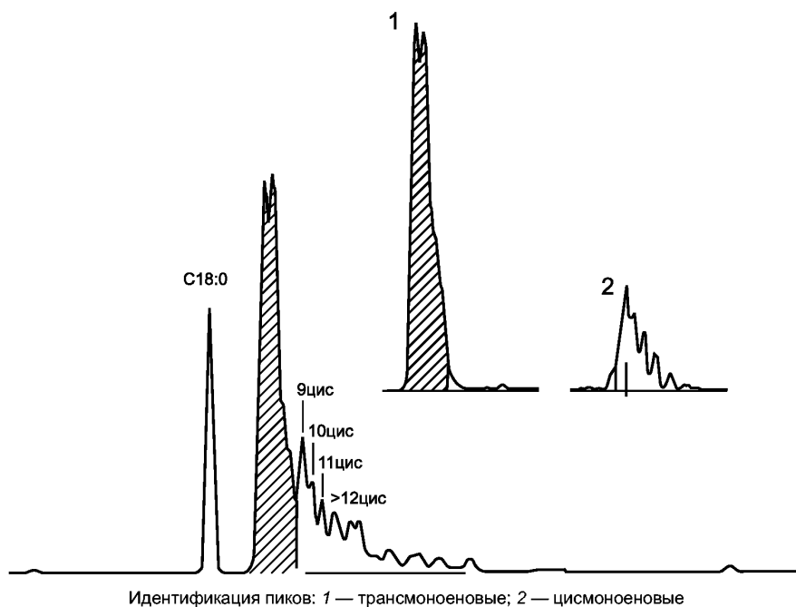
Рисунок Б.1 — Оптимальные условия для колонки типа ВРХ-70 при 198 °С (изотерма)
