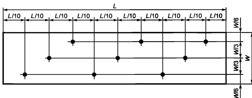
Рисунок 12 — Положение точек отбора проб на открытой поверхности железнодорожной платформы
