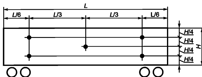
Рисунок 11 — Положение точек сбора проб на различных уровнях железнодорожной платформы
