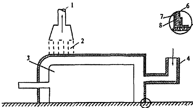
Рисунок 10 — Схема звукоизолирующего кожуха
