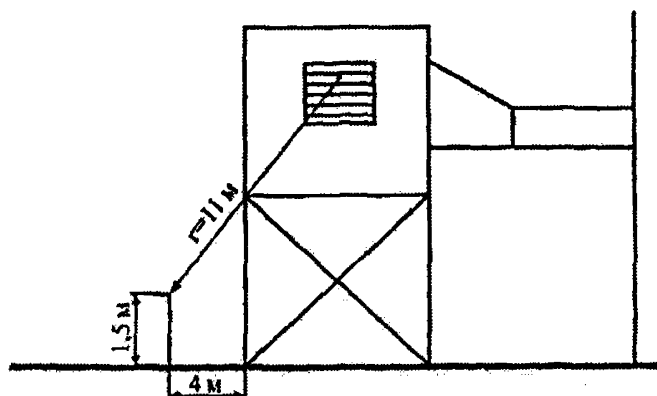
Рисунок 6 — Схема для акустического расчета глушителей шума всасывания
