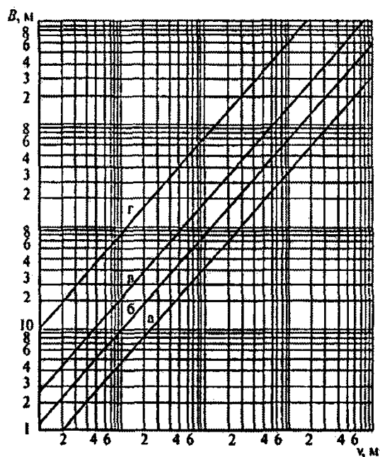
Рисунок 15 - Зависимость постоянной помещения B_{1000} от его объема V
