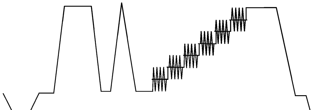
Рисунок 2 — Графическое изображение измерительного сигнала, содержащего сигнал Н1
