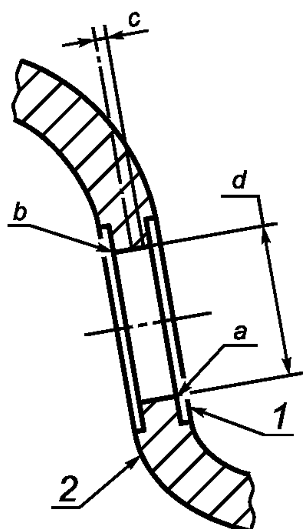
1 — сторона шины; 2 — наружная сторона a — см. 5.3.1.1; b — см. 5.3.1.2; c — см. 5.3.1.3; d — см. 5.3.1.4 Рисунок 7 — Вентильное отверстие обода
