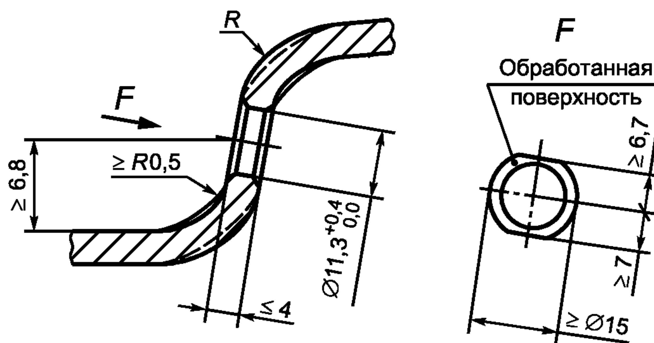
Рисунок 4 — Исполнение поверхности в зоне вентиляного отверстия
