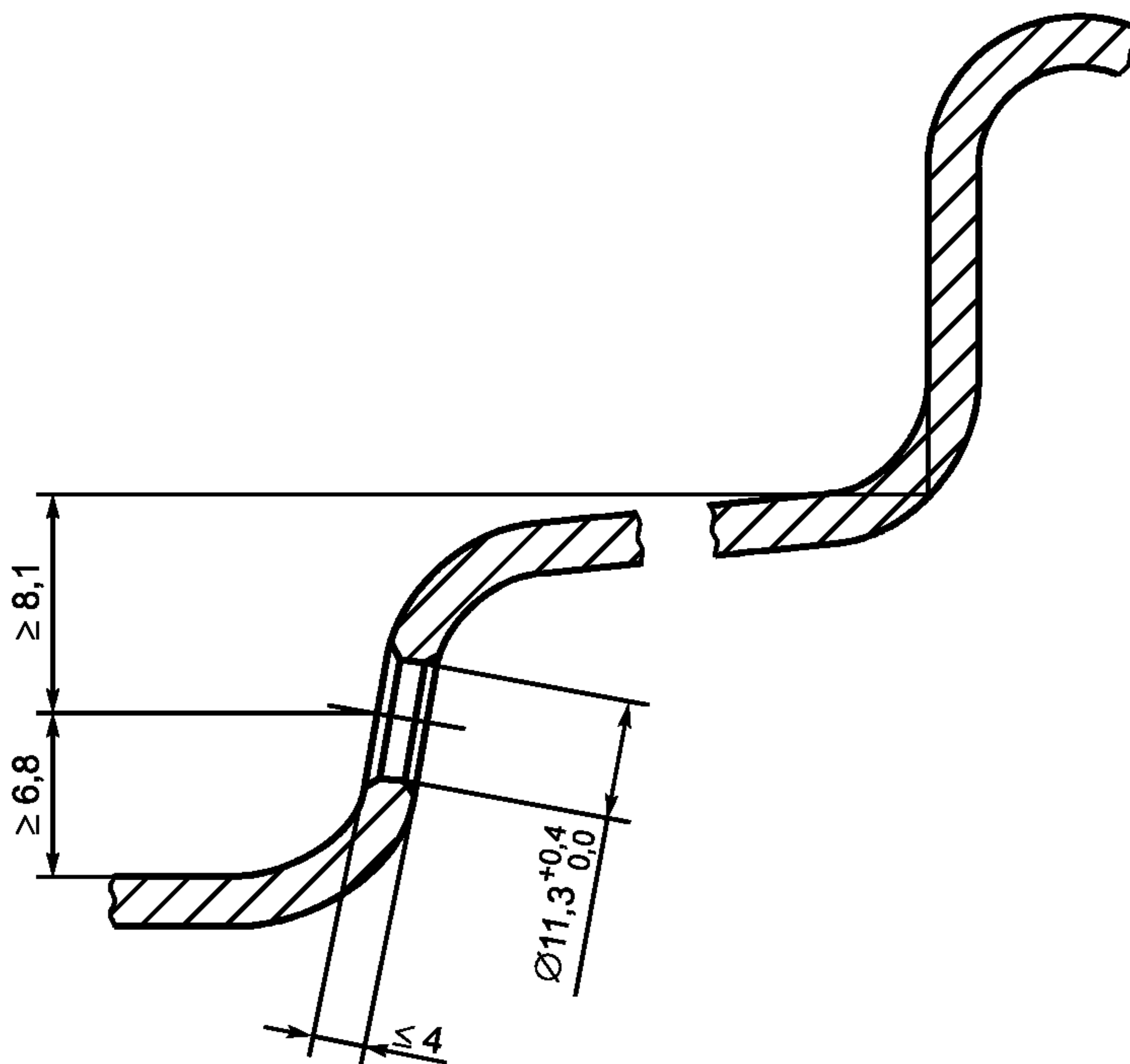
Рисунок 3 — Размеры вентиляного отверстия для бескамерных шин
