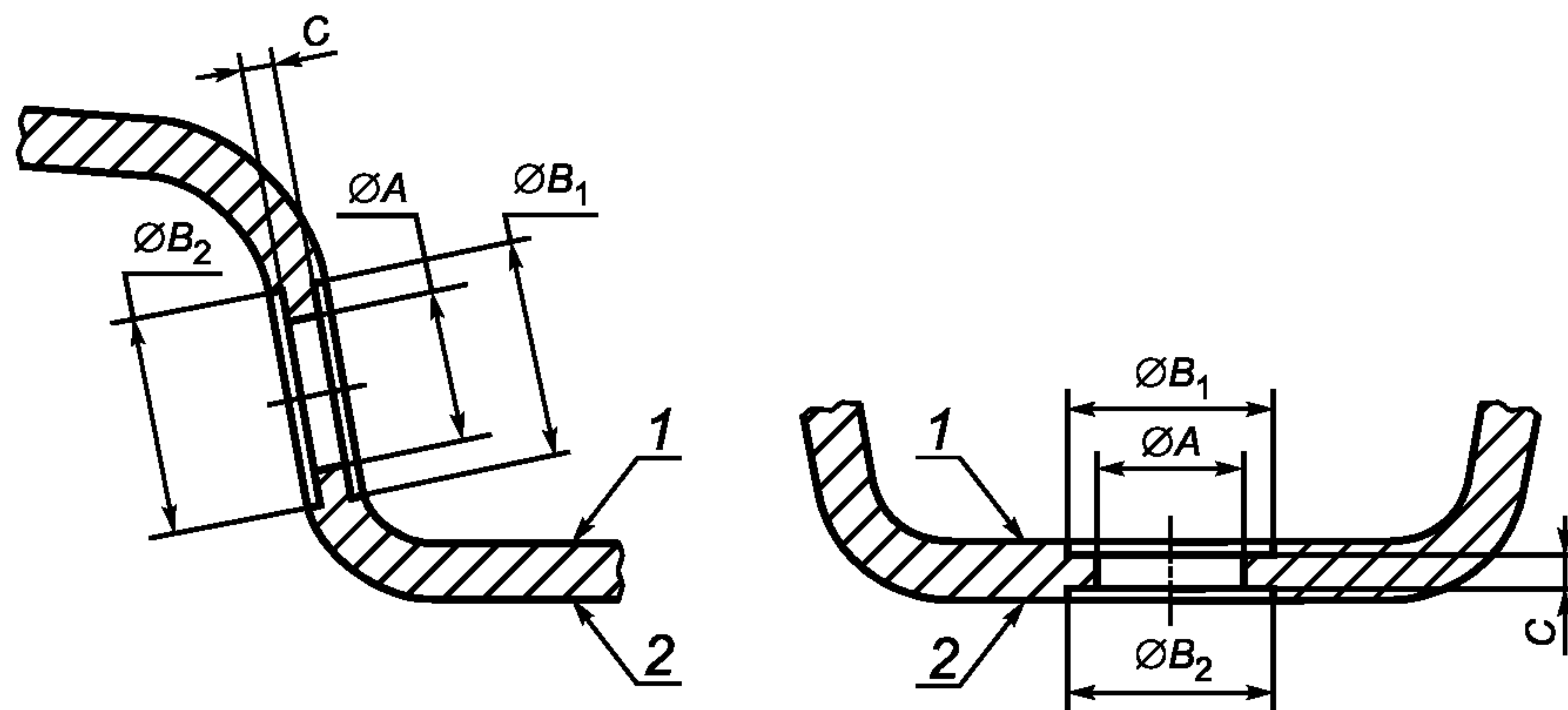
Боковая стенка монтажного ручья
