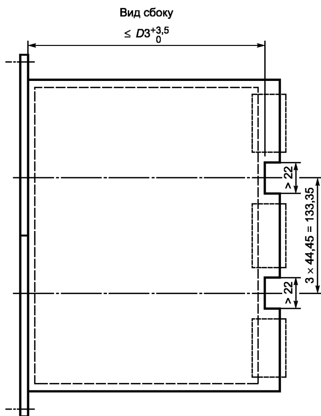
Рисунок 11 — Вставной блок с кожухом высотой 9U
