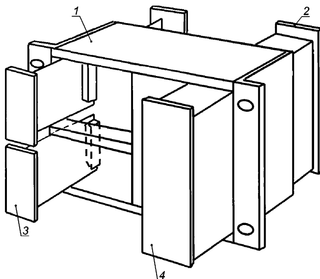
1 — типовой блочный каркас высотой 6U с возможностью вставки двух блоков размером 3U и одного 6U ; 2 — вставной блок высотой 6U в кожухе, устанавливаемый сзади; 3 — вставной блок высотой 3U в виде печатной платы, устанавливаемый спереди; 4 — вставной блок высотой 6U в кожухе, устанавливаемый спереди
