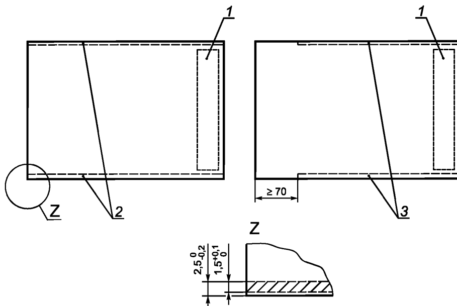
1 — зона соединителя; 2 — контактный элемент ЗЭР вдоль всей платы (с обеих сторон); 3 — контактный элемент ЗЭР прерван (с обеих сторон)
