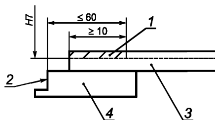
1 — расположение контактного элемента ЗЭР; 2 — плоскость закрепления переднего/заднего вставного блока; 3 — передняя/задняя направляющая блочного каркаса; 4 — передняя/задняя горизонтальная деталь
