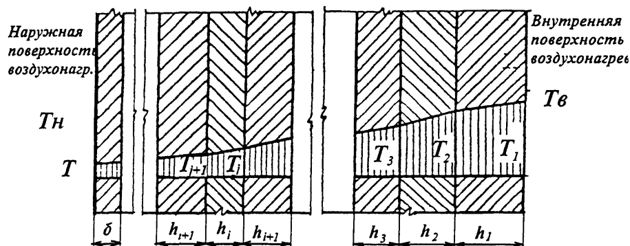
Рис. 7.5 Изменение температуры по толщине стенки воздухонагревателя
