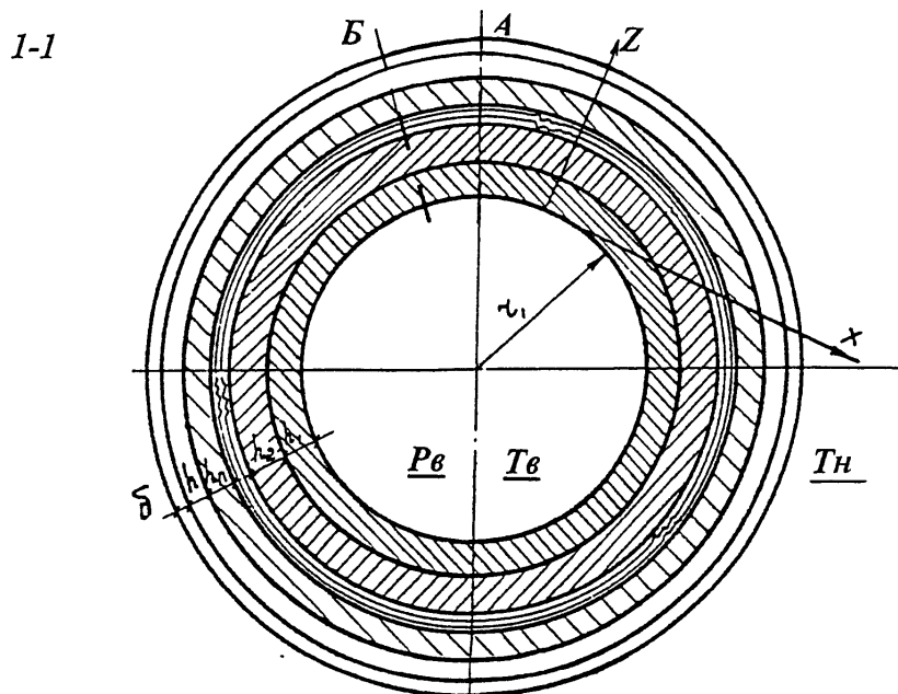
Рис. 7.10 Схема поперечного сечения 1-1
