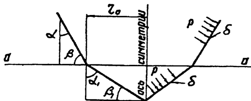
Рис. а Схема пересечения конусов
