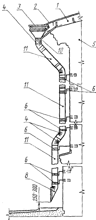
С применением звеньев труб типов ТВ1 и ТВ2
