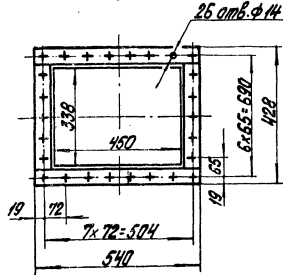
Фланец напорной патрубки дымохода и вентиллятора м 1:10
