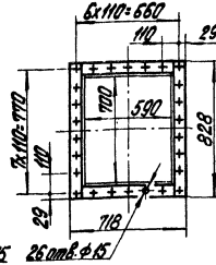
Фланец клапана 600 x 700 м 1:20
