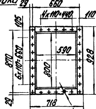
Фланец клапана 600 x 800 м 1:20
