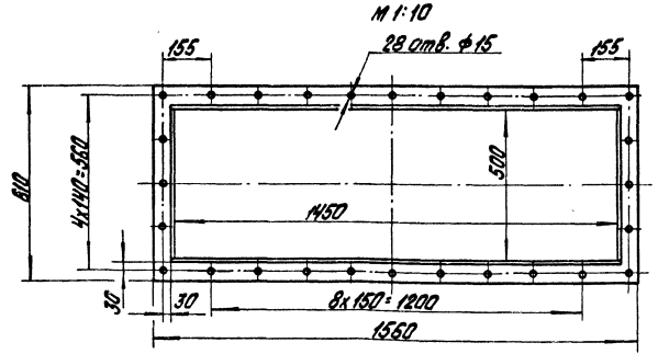
Входной фланец воздуха подогревателя м 1:10
