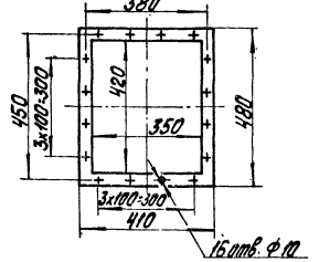
Выходной фланец воздуха подогревателя м 1:10
