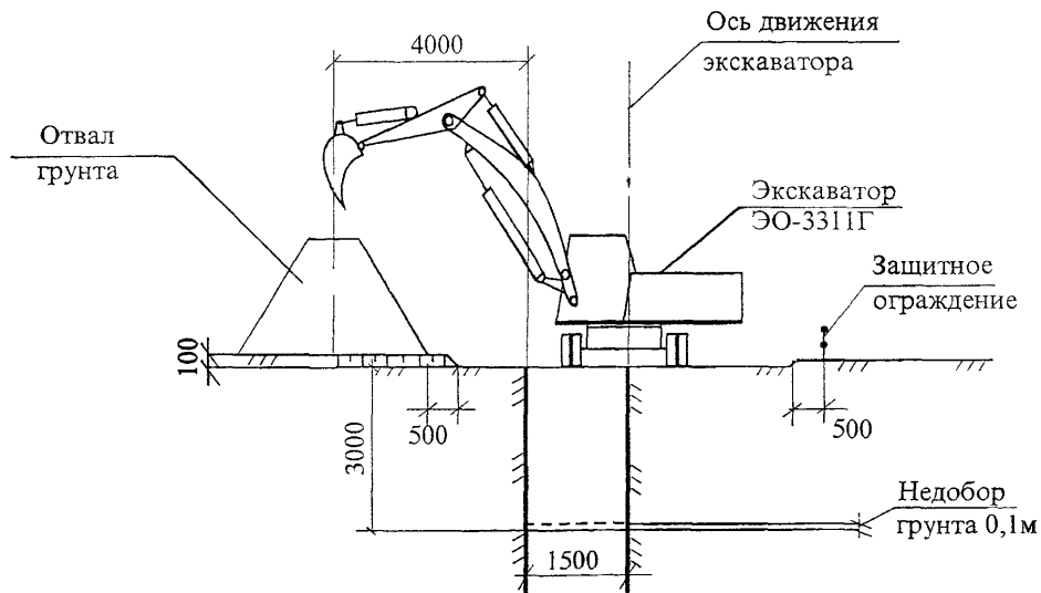
Рисунок 12 – Пример геометрии траншеи для цифровых расчетов
