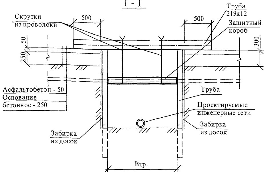
Рисунок 9 – Пример формирования траншей при пересечении с действующими коммуникациями
