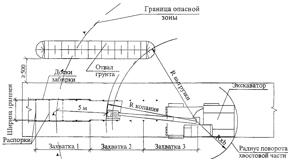
Рисунок 7 – Схема производства работ по разработке грунта траншеи экскаватором и устройства заборки
