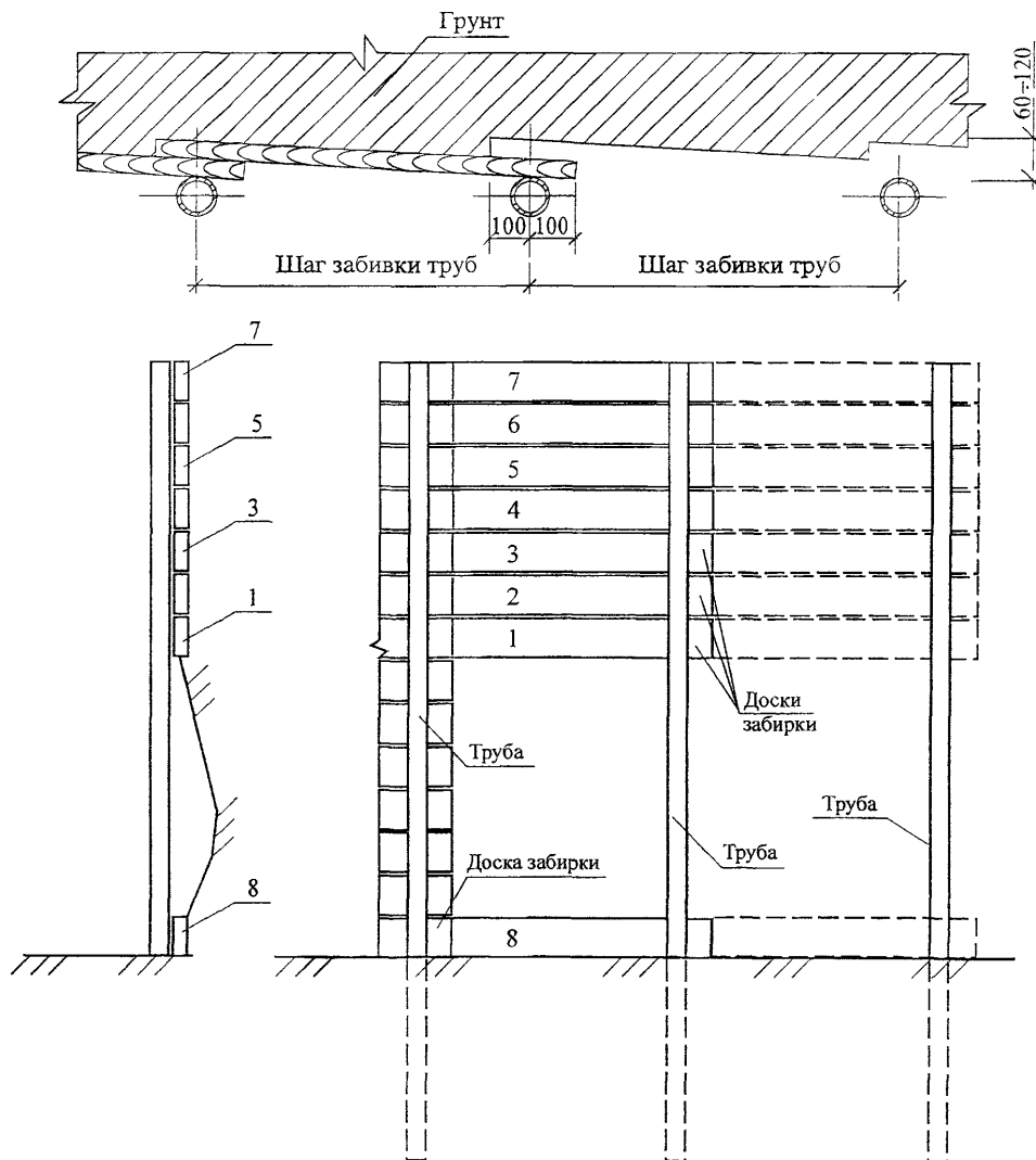
Рисунок 11 – Последовательность и схема устройства заборки
