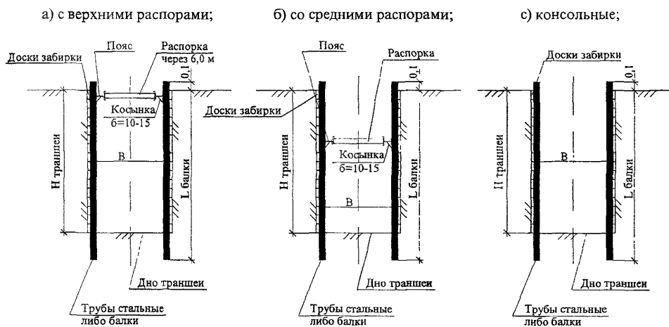
Рисунок 1 – Варианты крепления стенок траншей глубокого заложения
