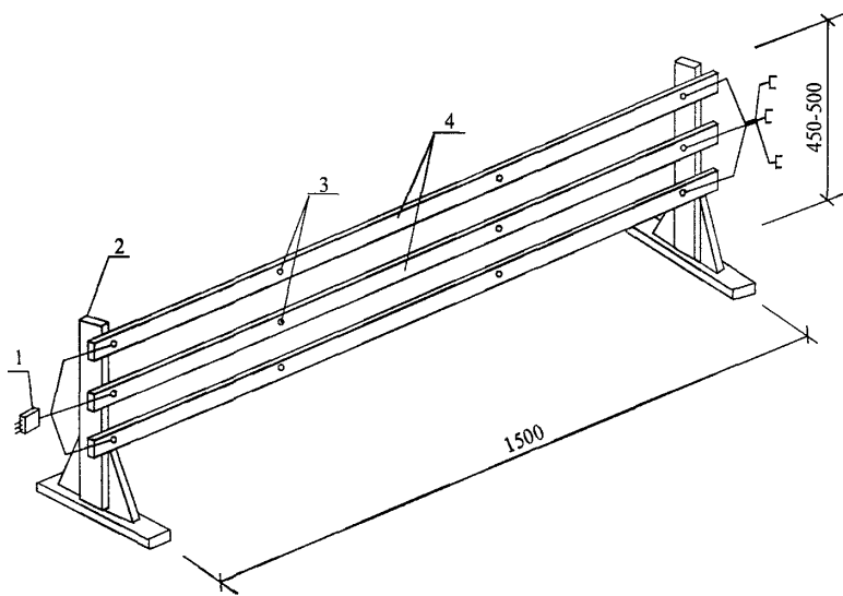
Рисунок 2 – Инвентарная секция шинопроводов (крайняя секция)
