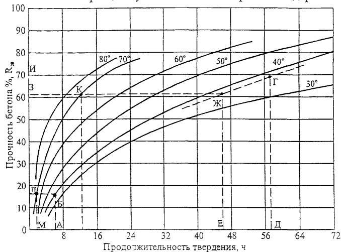
Рисунок 9 – Пример определения прочности бетона по графику
