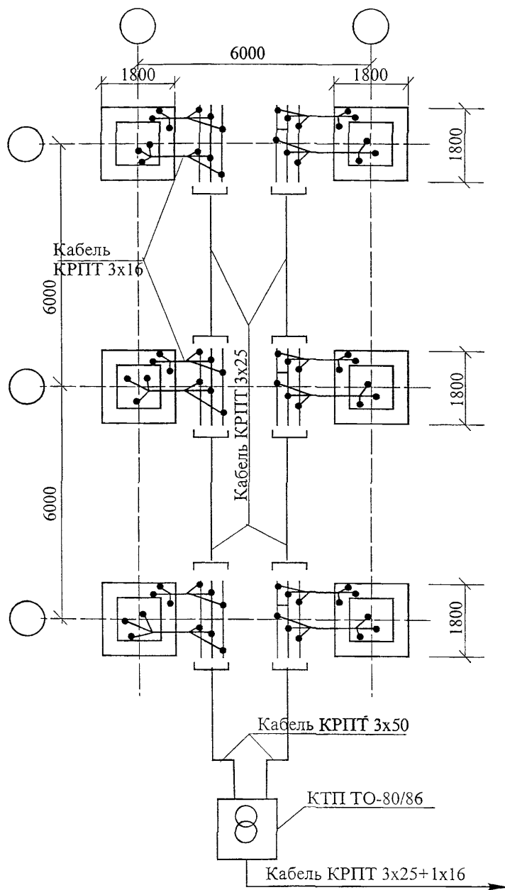
Рисунок 4 – Схема подключения шинопроводов к питающей сети
