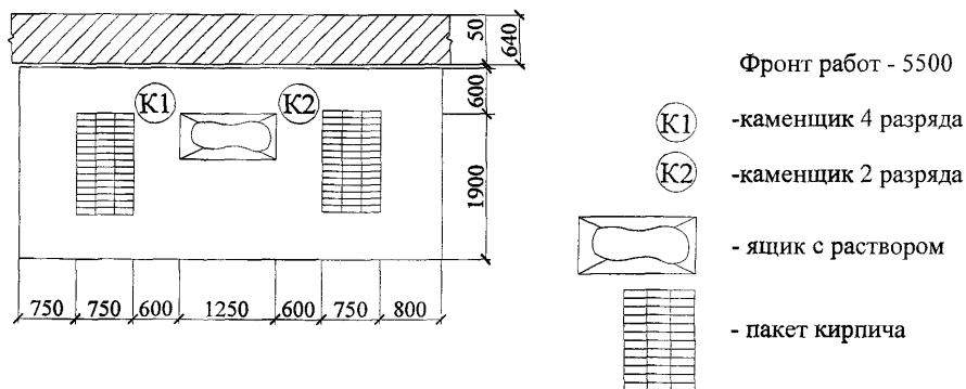
Рис.1 Рабочая зона звена
