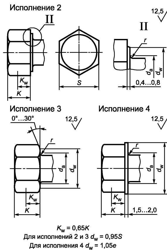
Рисунок А.2 — Конструктивное исполнение головки болта
