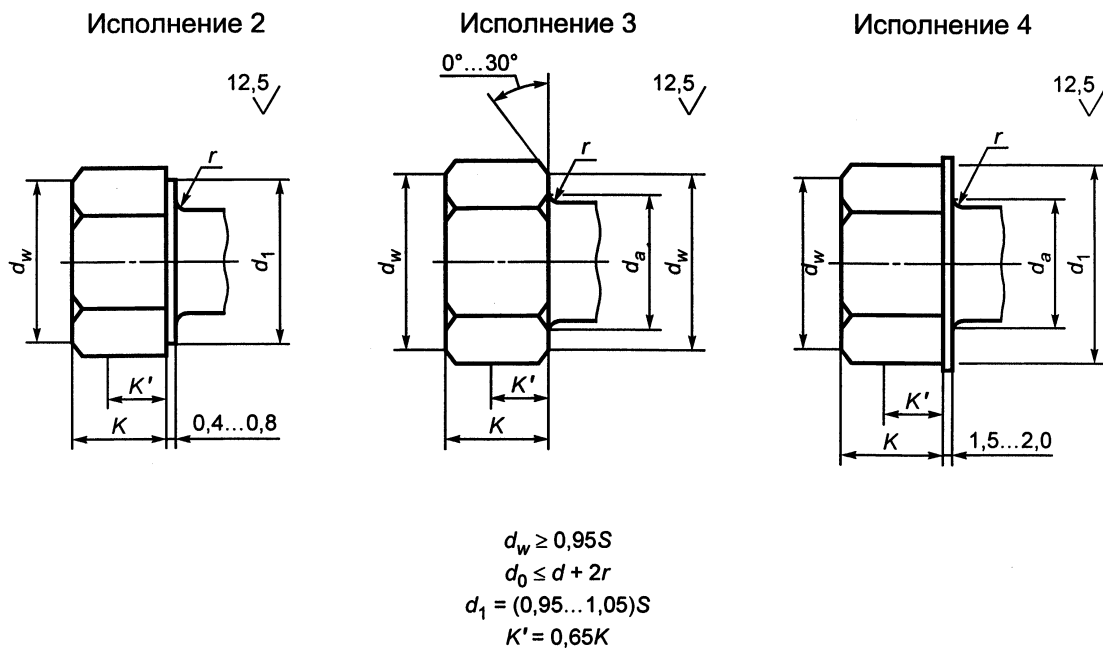
Рисунок А.2 — Конструктивное исполнение головки болта
