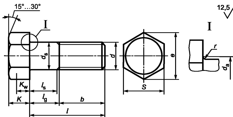
Рисунок 1 — Конструктивное исполнение тела болта 1 (основное исполнение)
