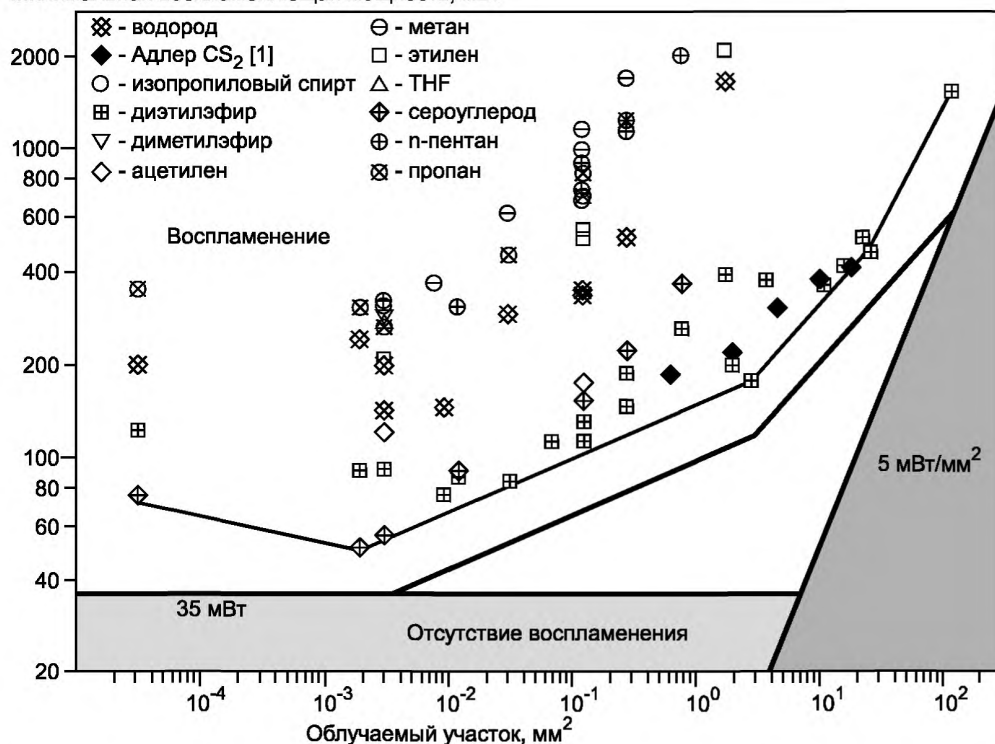
Рисунок 1 — Рисунок В.1 с предельными линиями для промежуточных значений площадей облучаемой поверхности в присутствии негорючих поглотителей (классы температур T1—T4, электрооборудование подгрупп IIA, IIB, IIC)
