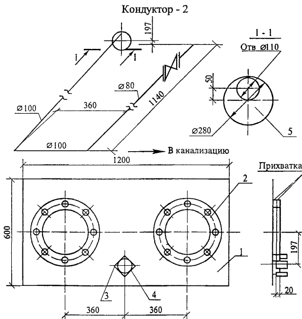
Рисунок 4 – Узел подвода воды к форсункам
