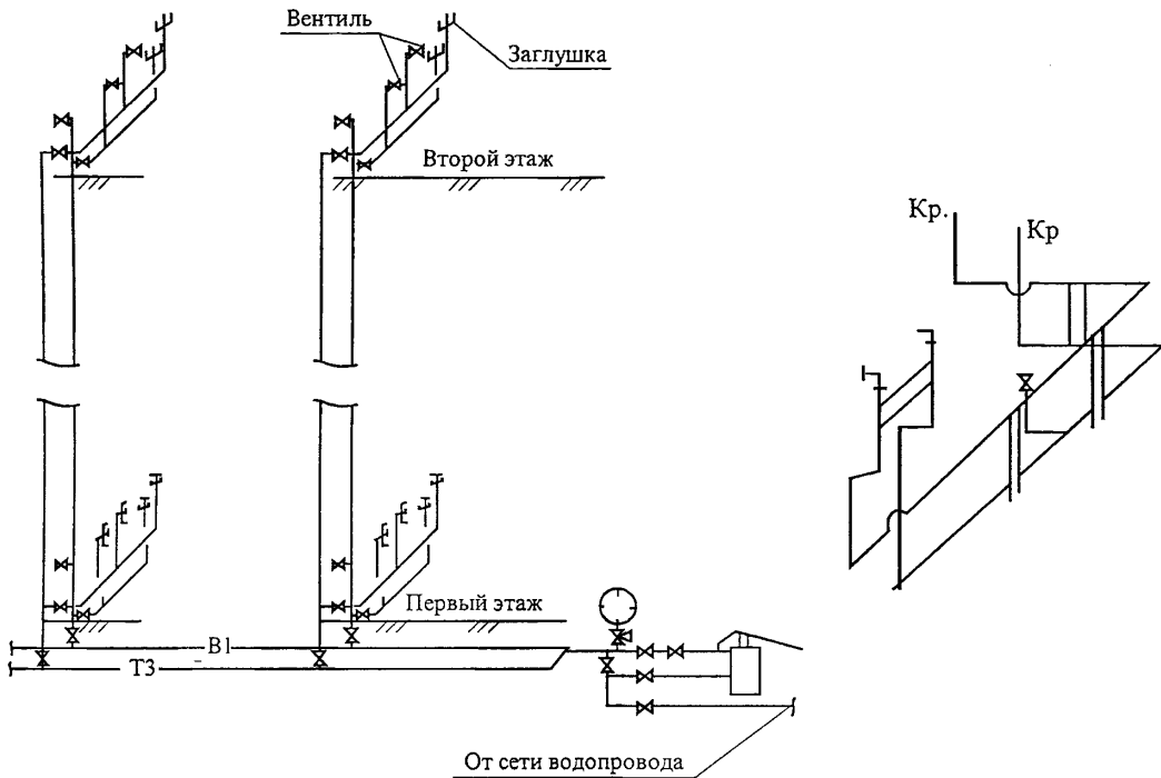
Горизонтальный блок
