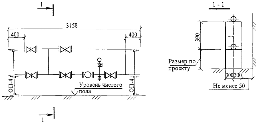
Рисунок 1 – Схема установки водомерного узла № 12
