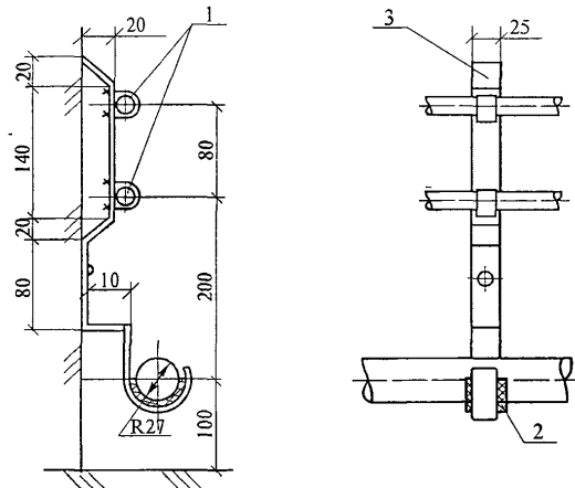
Рисунок 7 – Кронштейны для крепления трубопровода горизонтального блока
