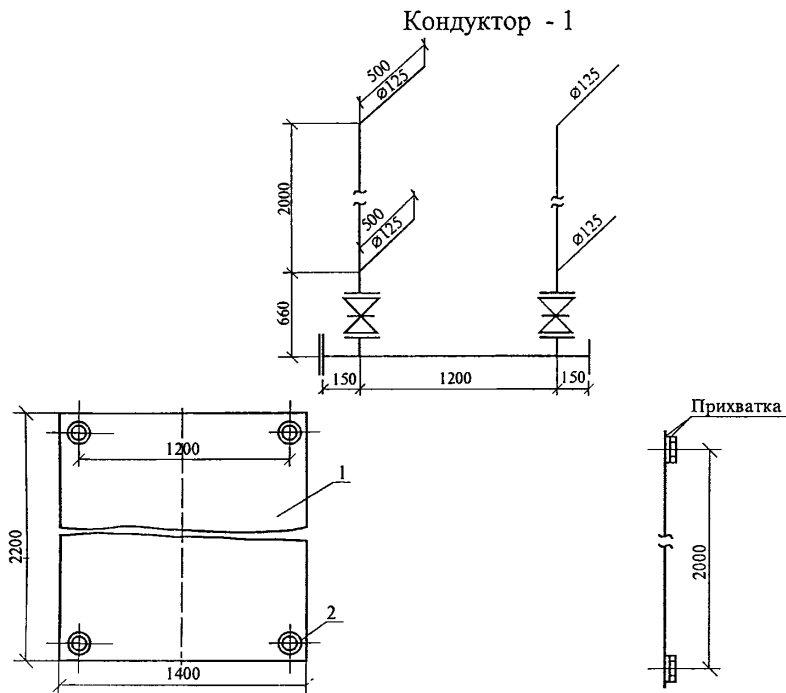
Рисунок 4 – Узел подвода воды к форсункам
