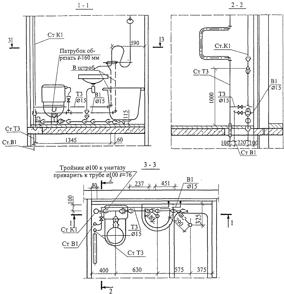
Рисунок 2 – Совмещенный санузел типа ЗСУ пр 02
