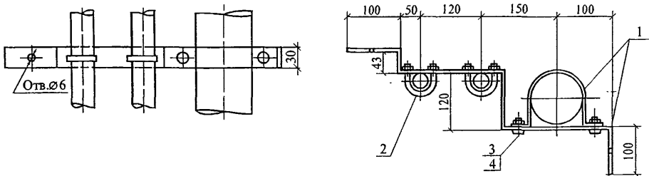
Рисунок 7 – Кронштейны для крепления трубопровода горизонтального блока
