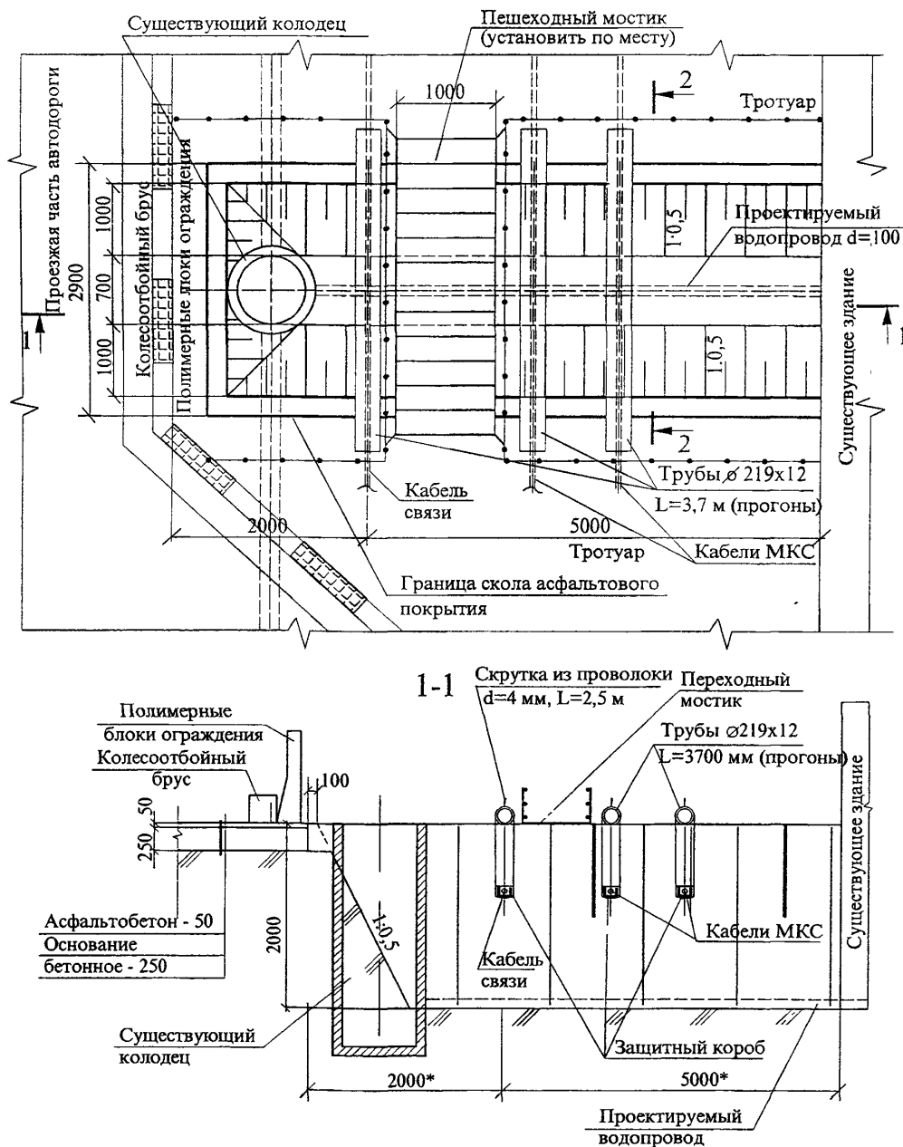
Рисунок 6 – Примерная схема пересечения трубопровода с кабелями связи и МКС
