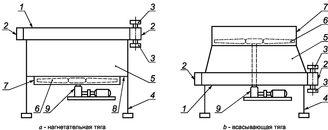
Рисунок 2 — Типичные элементы аппарата с воздушным охлаждением
