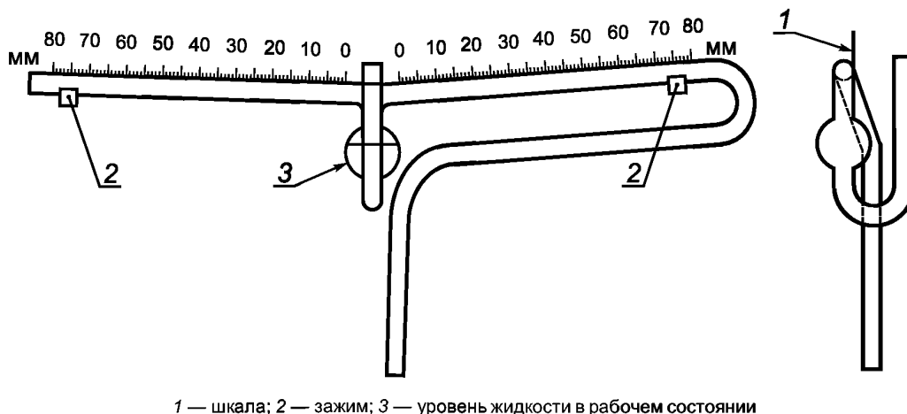
Рисунок F.4 — Трубка Парджо (тип А)
