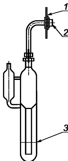
1 — панель; 2 — направление от НЕРА фильтра; 3 — уровень масла
