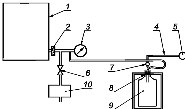
1 — изолирующее устройство; 2 — НЕРА фильтр (опция); 3 — манометр; 4 — резиновая трубка; 5 — пипетка; 6 — изолирующий вентиль; 7 — трубка Парджо; 8 — резиновая пробка; 9 — изолированный стеклянный сосуд; 10 — источник давления или вакуума
