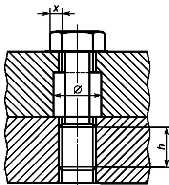
Рисунок 2 — Допуски и зазор для нарезных крепежных деталей
