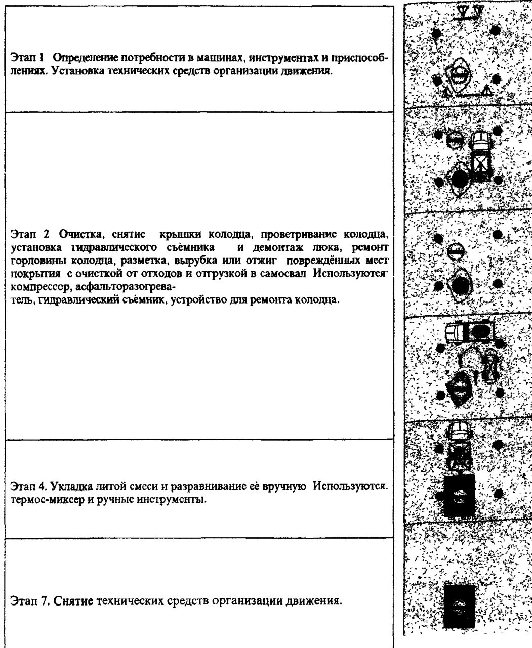
Рис.11. Технологическая схема ремонта асфальтобетонного покрытия у люка смотрового колодца литой асфальтобетонной смесью.
