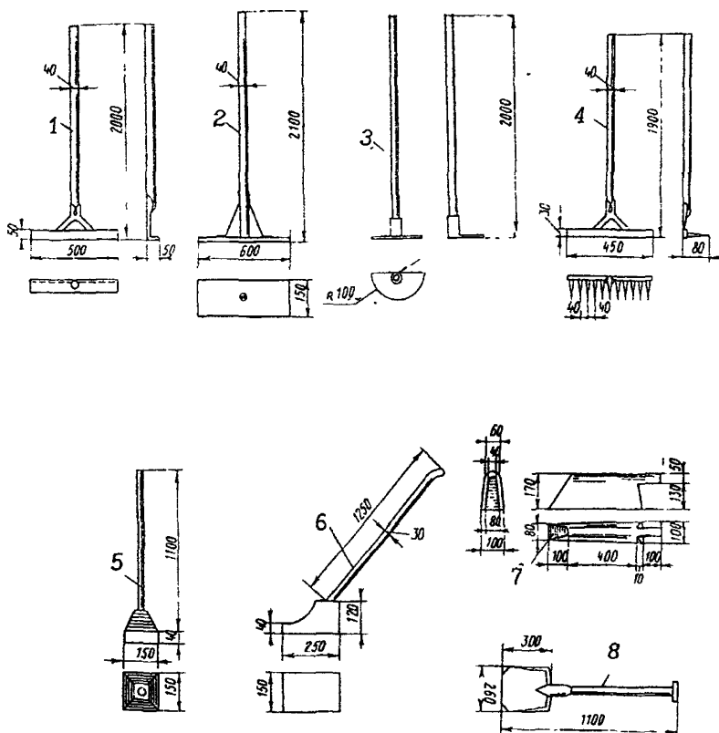
Рис. 6. Ручные инструменты для укладки литой асфальтобетонной смеси.
