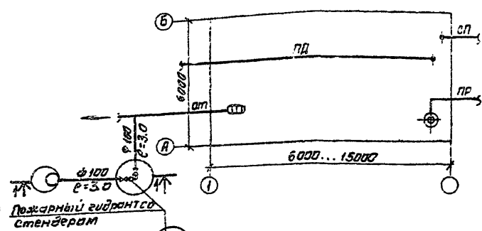
План резервуара емк. 5000...10000 м 3
