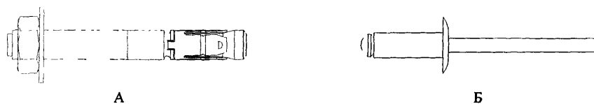
Рис.Б.11. Стальной анкерный дюбель (анкер) (А), заклепка вытяжная (Б).
