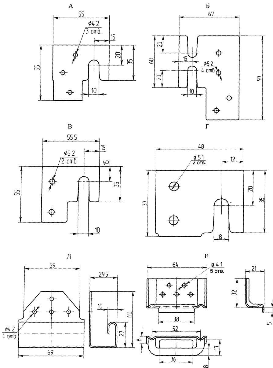
Рис.Б.5. Детали крепления облицовочных панелей (кассет): скоба универсальная SKU (А), скоба концевая СКК (Б), скоба рядовая СКР (В), скоба СКН (Г), зацеп ОЗ-1 (Д), зацеп ОЗ-3 (Е).
