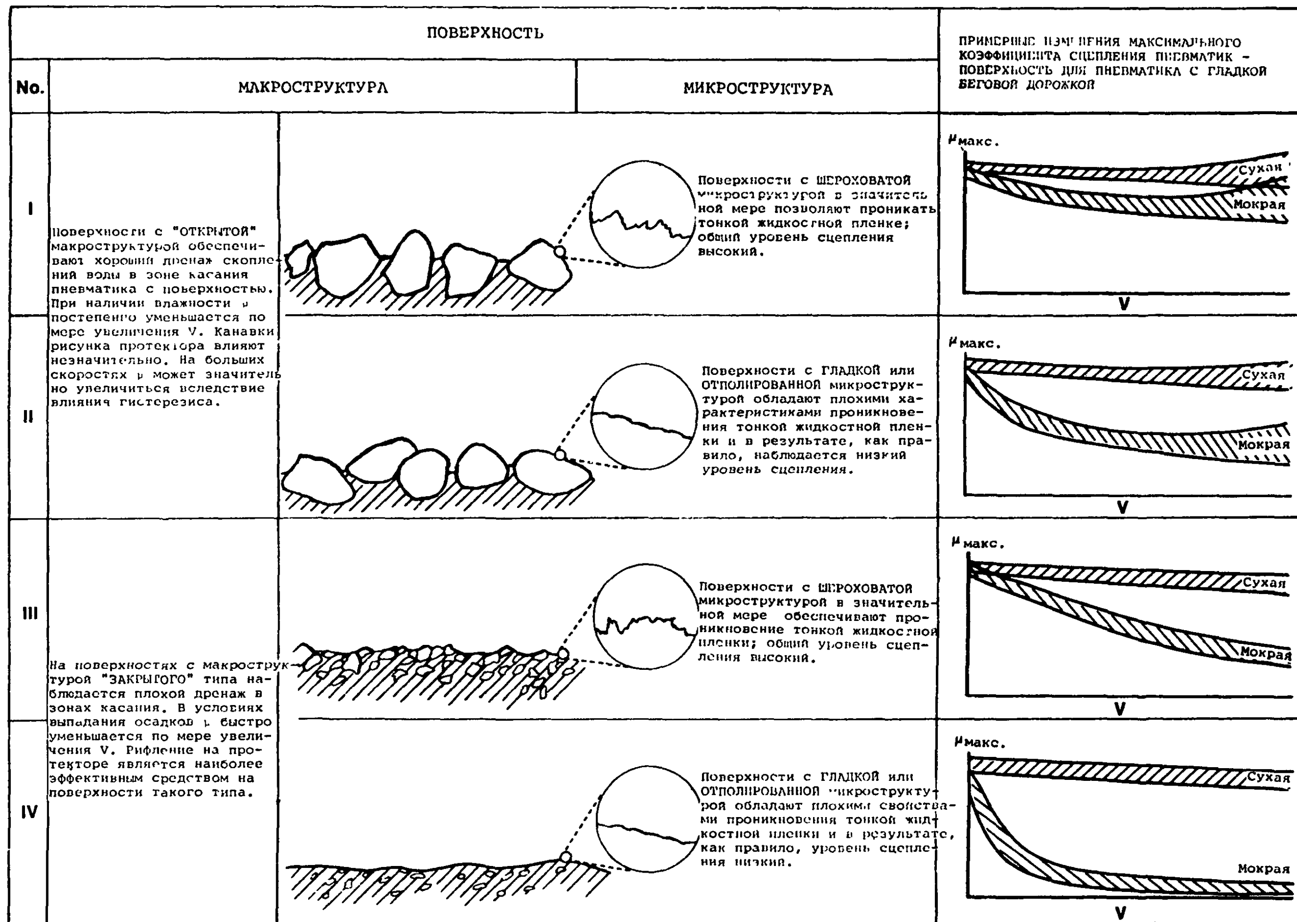
Рис. 5-2. Воздействие структуры поверхности на коэффициент сцепления пневматик-поверхность
