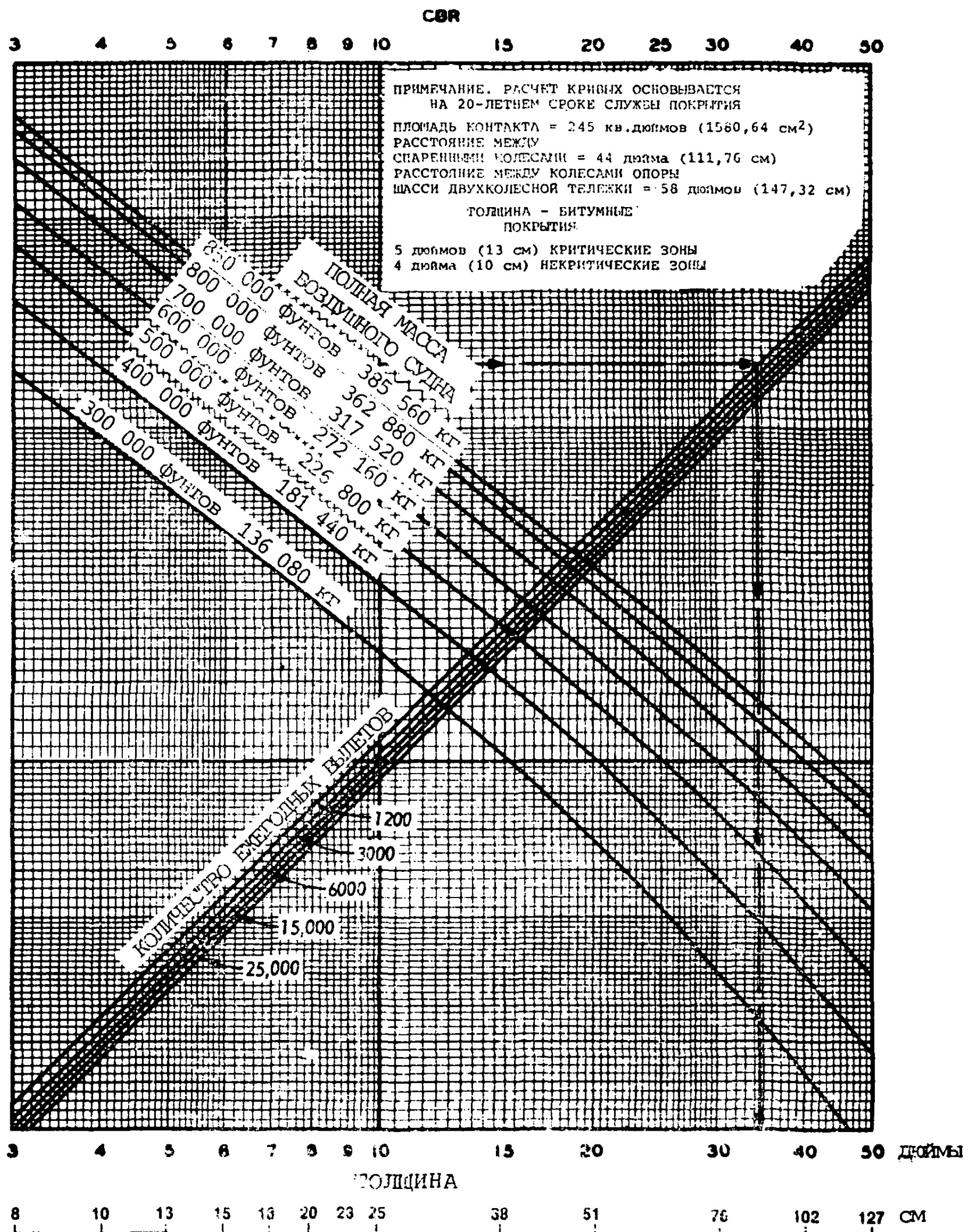
Рис. 4-39. Расчетные кривые нежестких покрытий для критических зон - В-747-100, SR, 200 В, С, F
