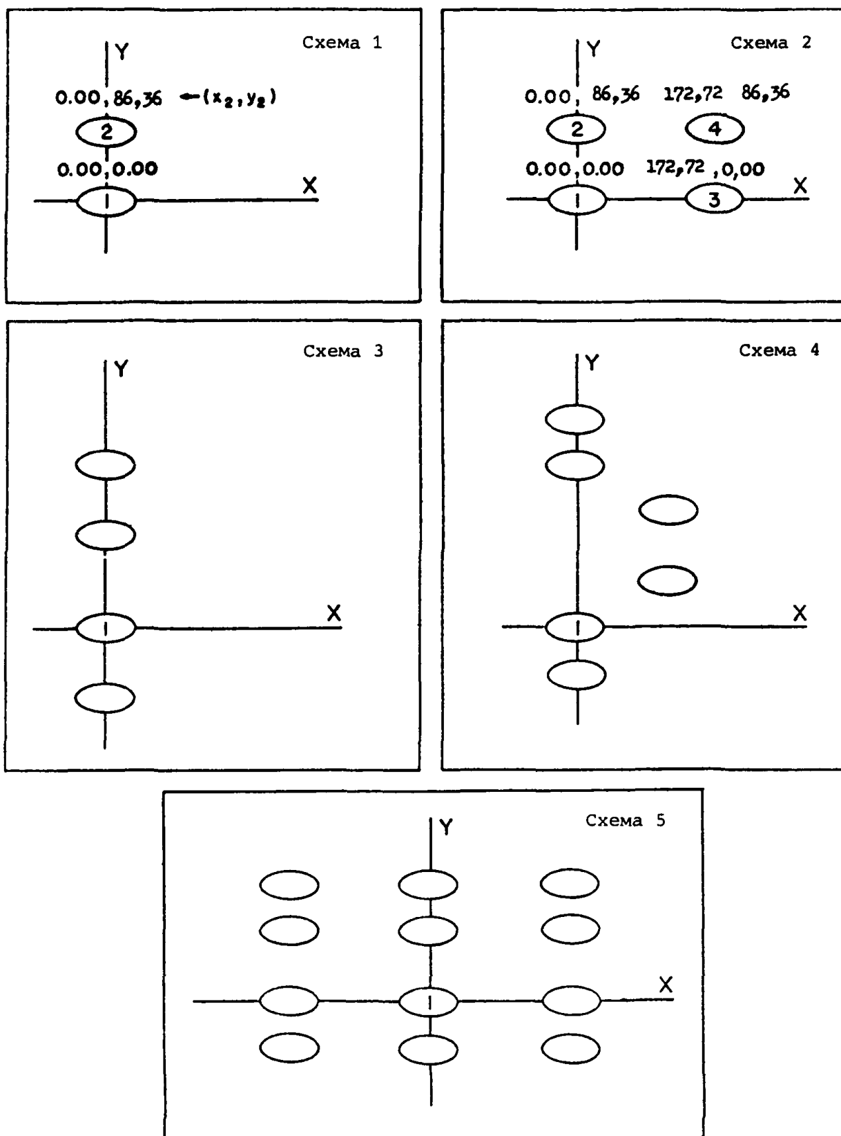
Рис. А2-2. Координаты колес и выбор колеса 1
