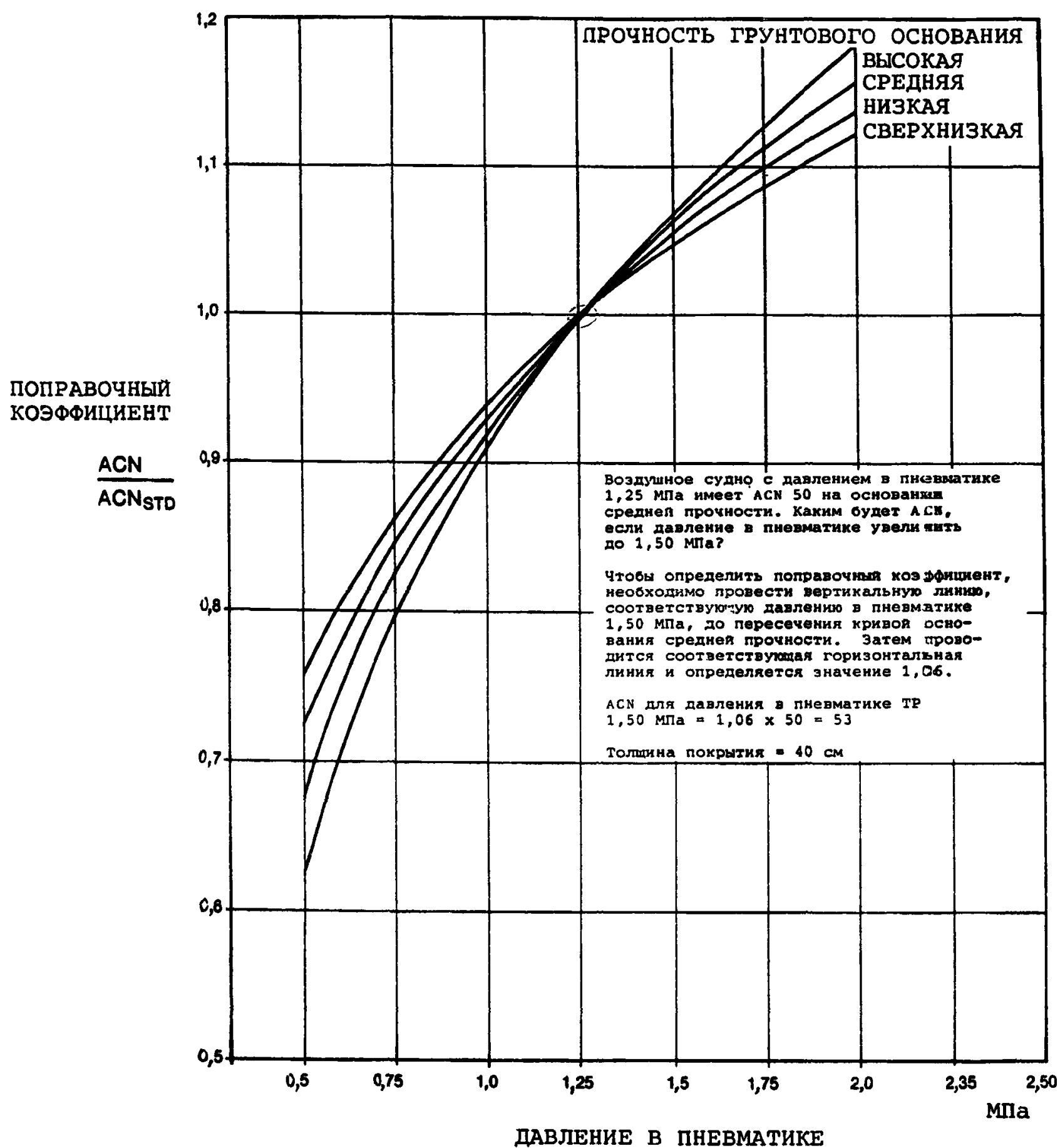
Рис. 1-6. Корректирование ACN по давлению в пневматике - только на жестком покрытии
