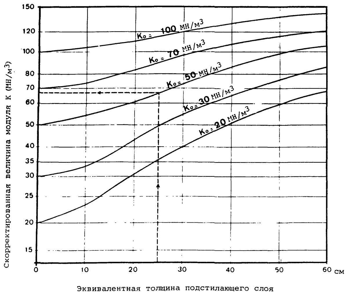
Рис. 3-13. Модуль реакции подстилающего слоя. Коррекция модуля реакции грунтового основания на основе эквивалентной толщины подстилающего слоя
