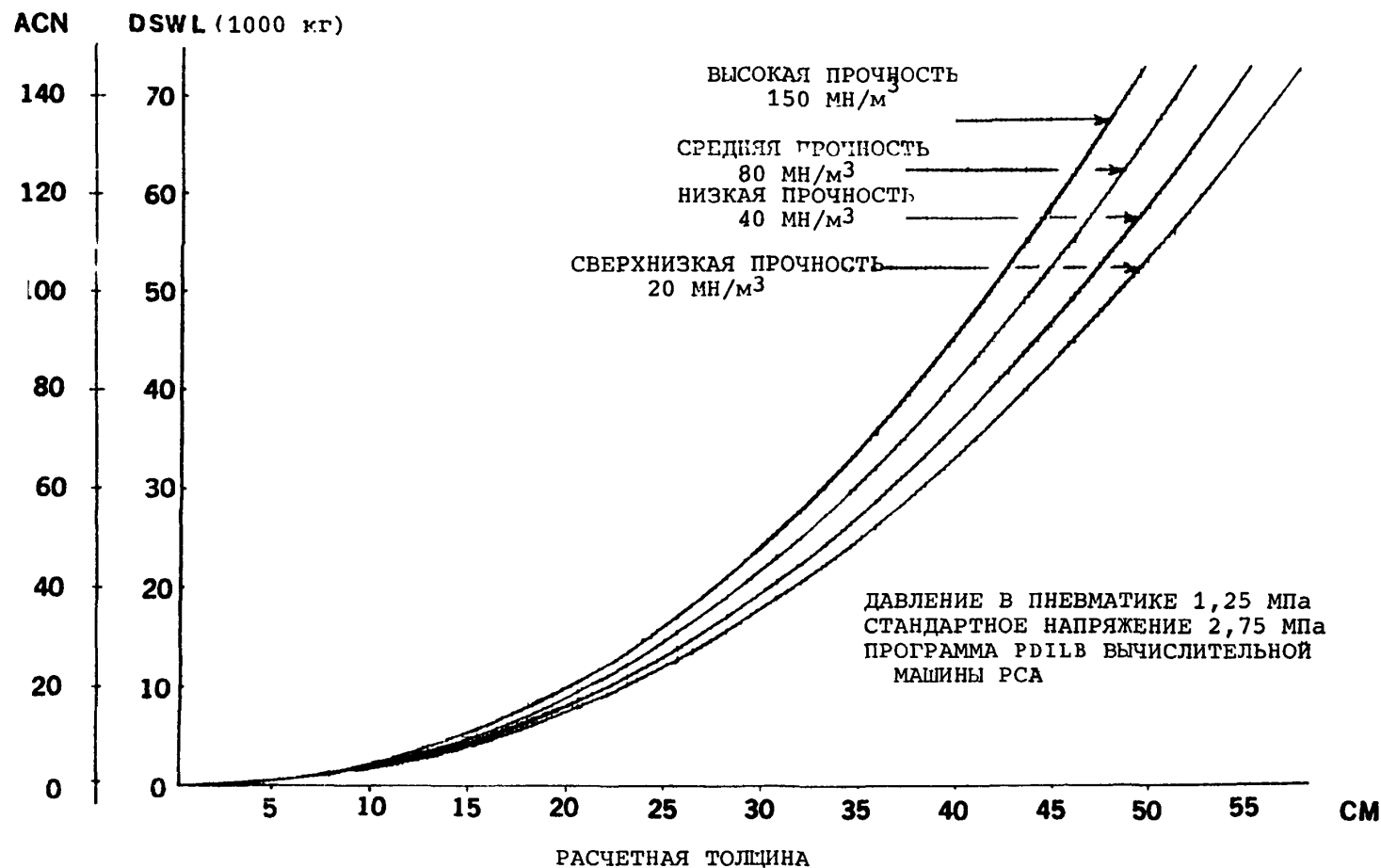
Рис. 1-4. График пересчета ACN на жестком покрытии
