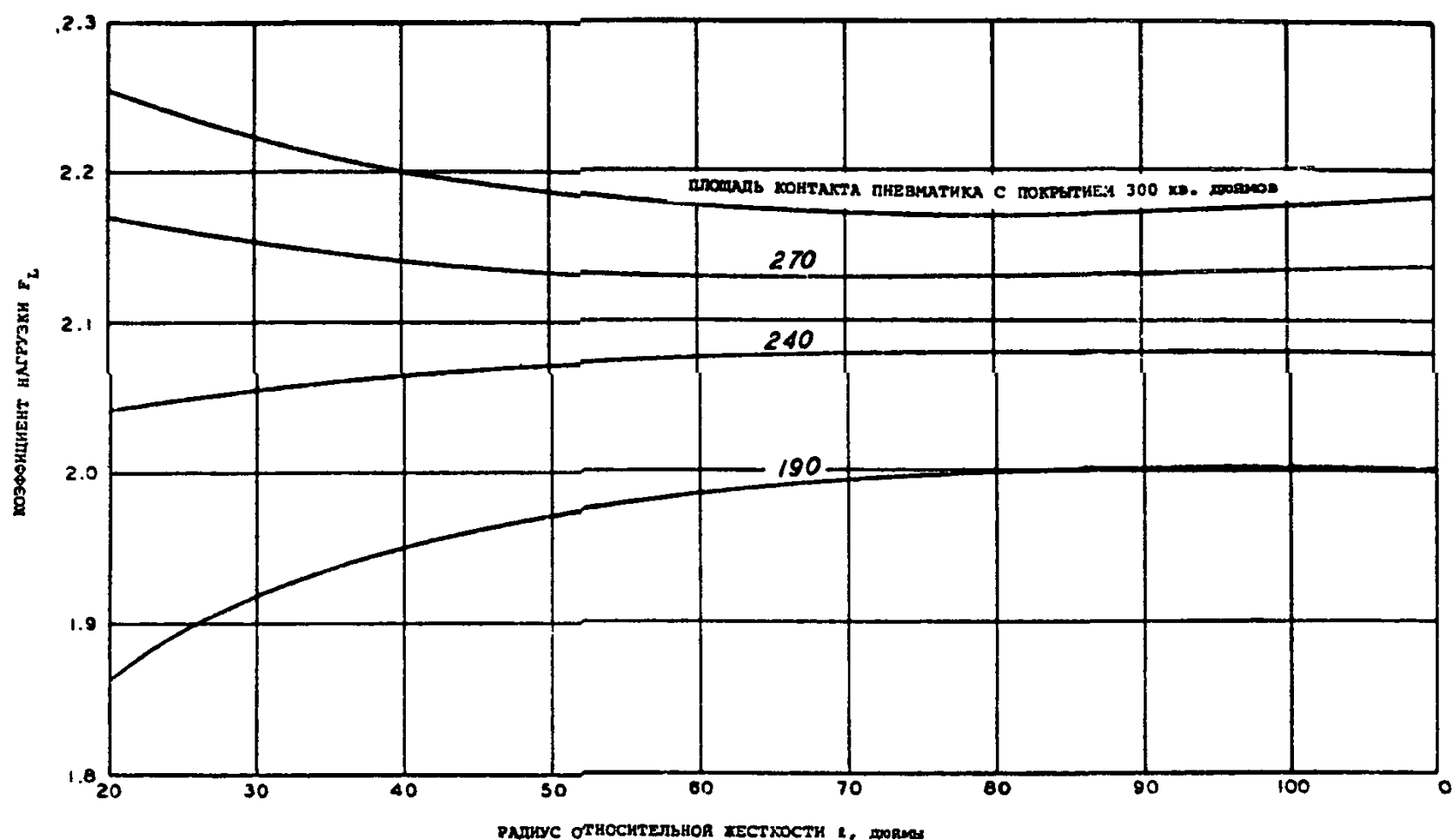
Рис. 3-11. Зависимость между F_L и l для воздушных судов с одноколесными опорами шасси на жестком покрытии
