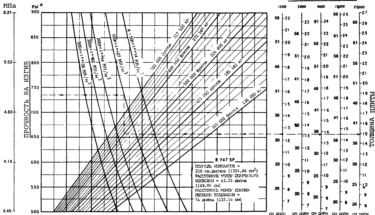
Рис. 4-50. Расчетные кривые жестких покрытий - В-747-SP
