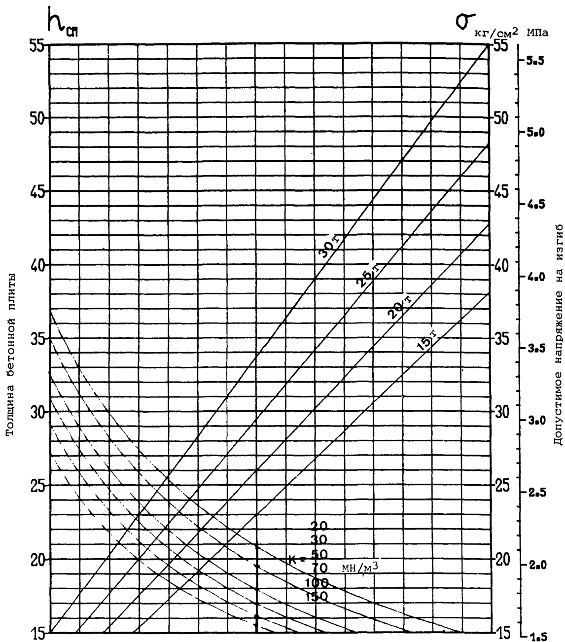
Рис. 4-24. Жесткое покрытие - типовая опора шасси - четырехколесная тележка Нагрузки от 15 до 30 тонн
