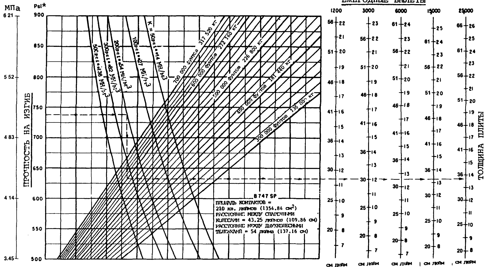
Рис. 4-58. Нестандартные расчетные кривые жестких покрытий - B-747-SP
