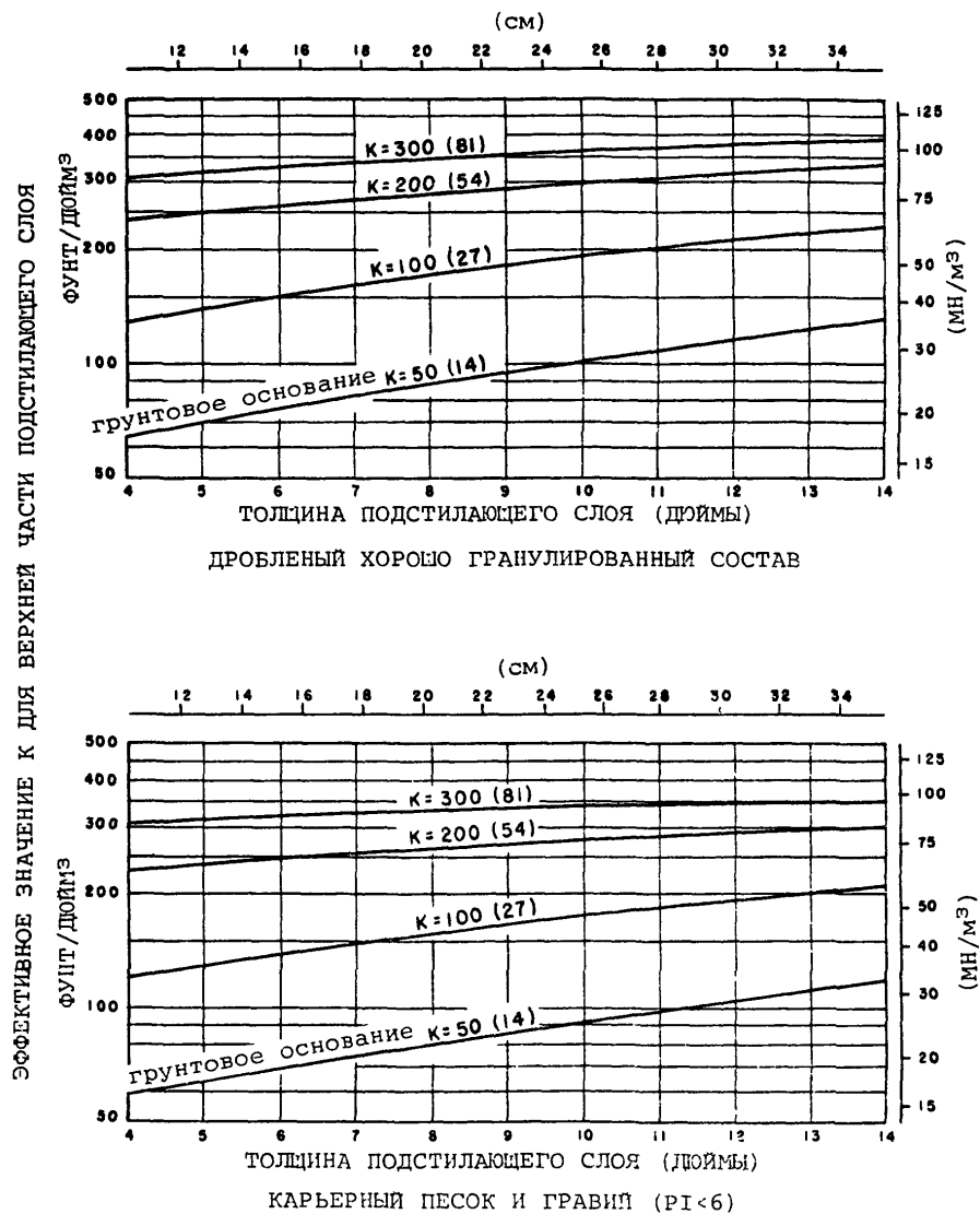
Рис. 4-35. Влияние подстилающего слоя на модуль реакции грунтового основания
