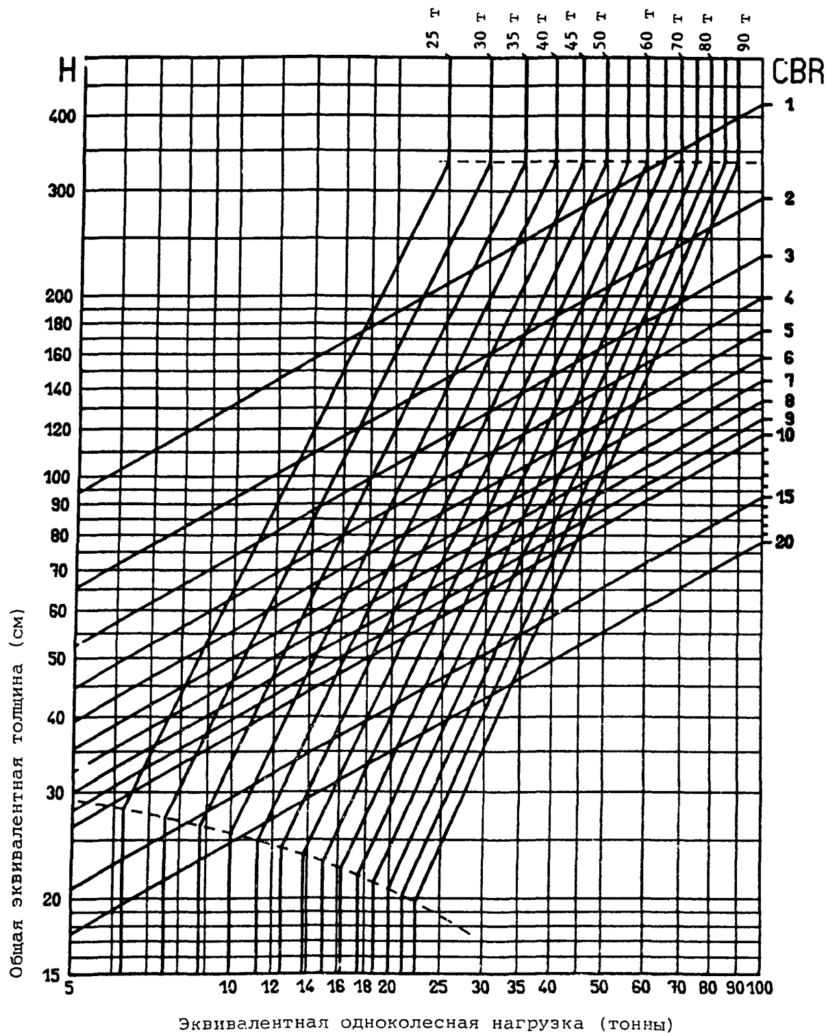
Рис. 4-17. Нежесткое покрытие - типовая опора шасси - четырехколесная тележка
