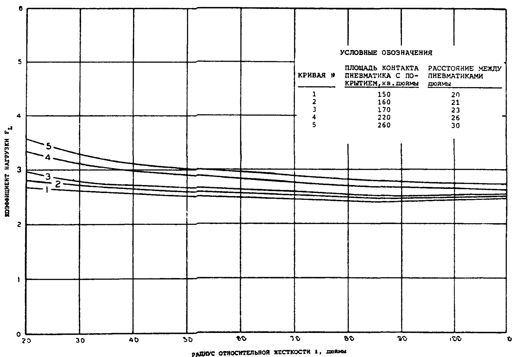
Рис. 3-11. Зависимость между F_L и l для воздушных судов с одноколесными опорами шасси на жестком покрытии
