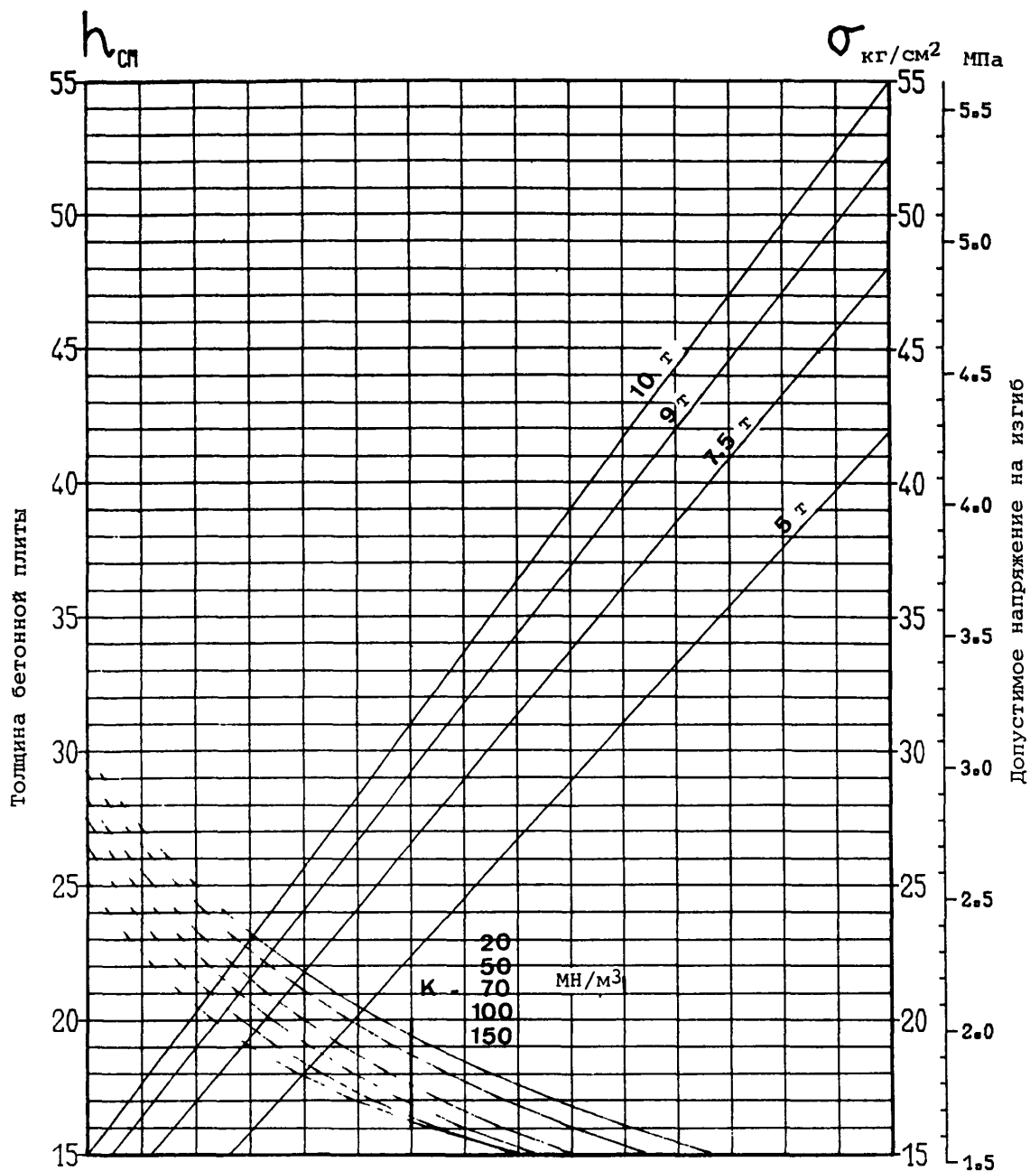
Рис. 4-18. Жесткое покрытие - типовая опора шасси - одиночное изолированное колесо Нагрузки менее 10 тонн
