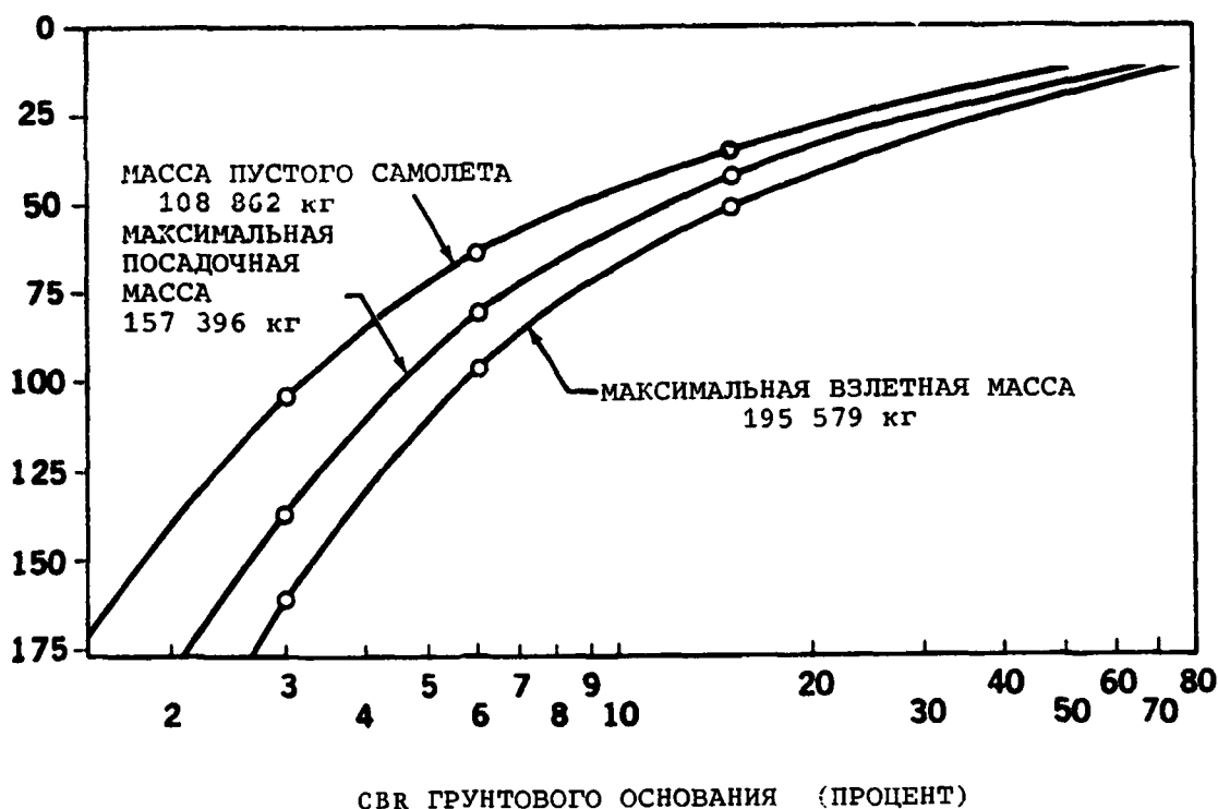
Рис. 1-8. Требования ДС-10-10 к нежесткому покрытию 10 000 проходов воздушных судов с хвостовым центром тяжести по полосе охвата
