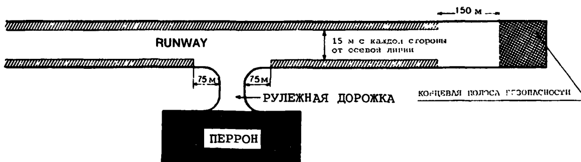
б) Пример ВПП, не оборудованной параллельными рулежными дорожками
