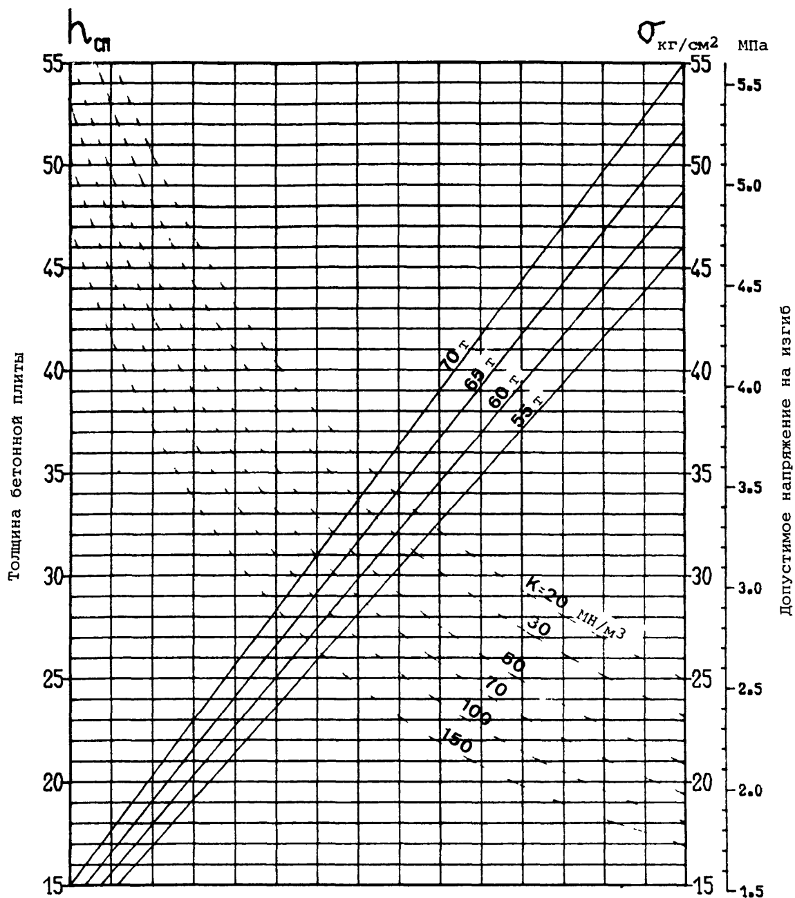
Рис. 4-26. Жесткое покрытие - типовая опора шасси - четырёхколесная тележка Нагрузки от 55 до 75 тонн
