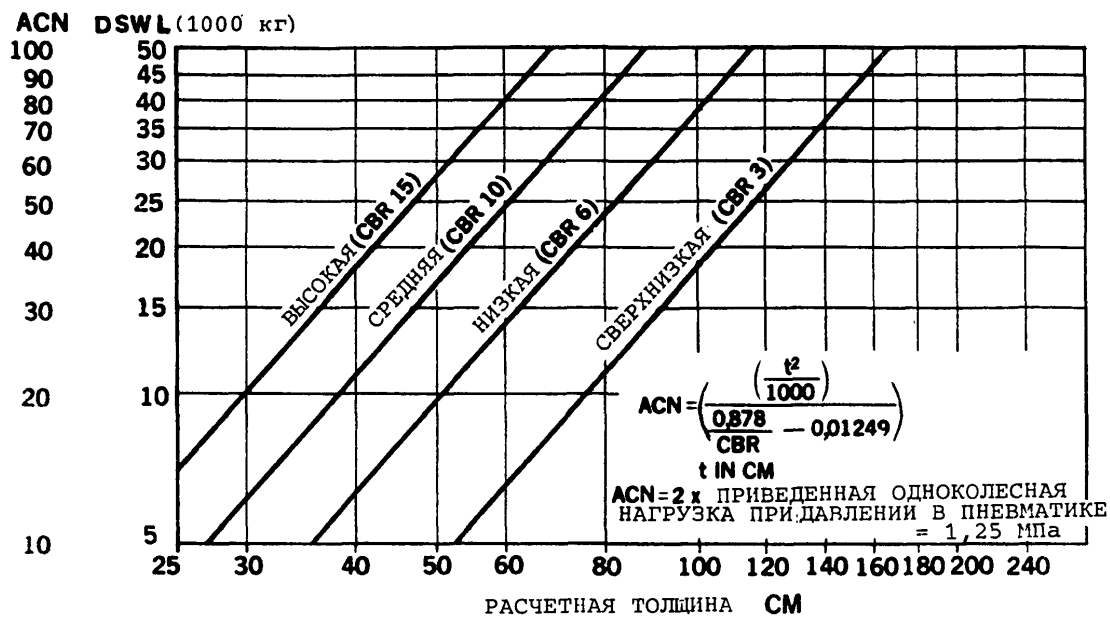
Рис. 1-5. График пересчета ACN на нежестком покрытии
