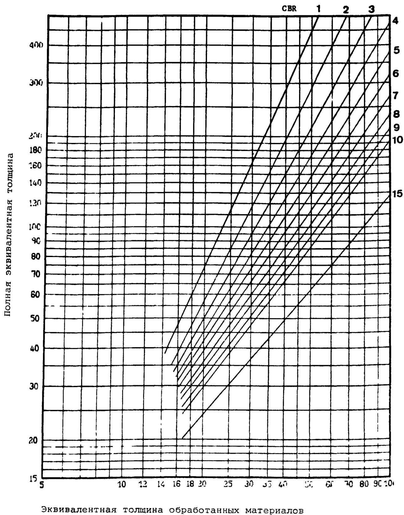
Рис. 4-12. Нежесткие покрытия: оптимальная толщина обработанных материалов по отношению к эквивалентной толщине обработанных материалов, полной толщине покрытия и величине СБР
