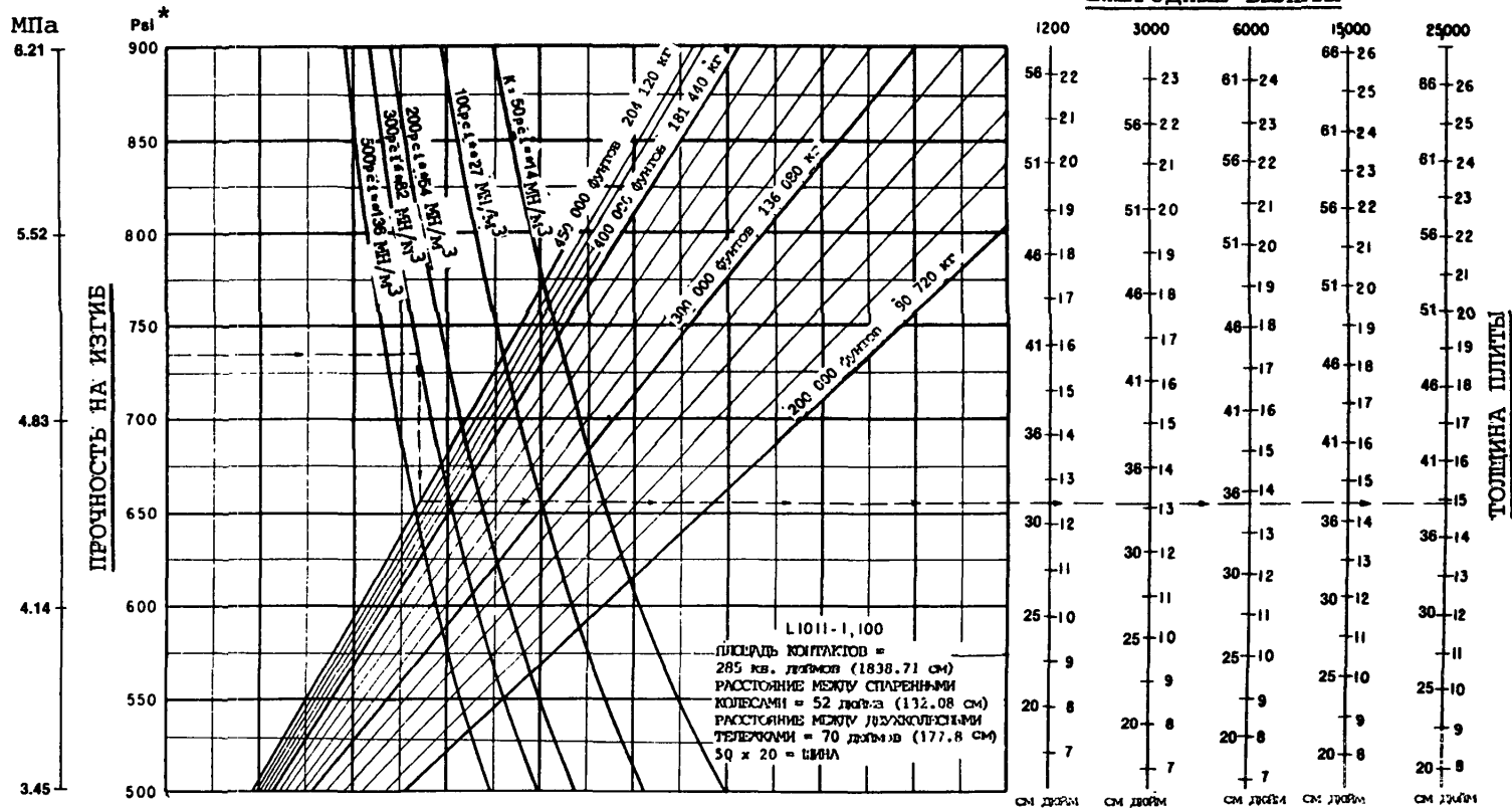
Рис. 4-61. Нестандартные расчетные кривые жестких покрытий - L-1001-1, 100
