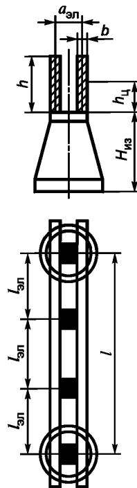
Рисунок 4 — Двухполосная шина
