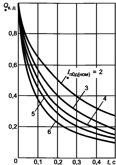
Рисунок 18 — Кривые для определения Q_{к.д} от асинхронного электродвигателя
