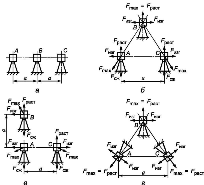
Рисунок 2 — Схемы взаимного расположения шинных конструкций
