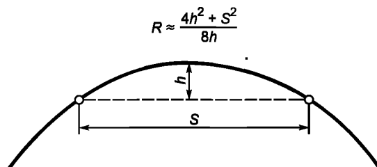
Рисунок 2 — Схема определения радиуса горизонтальной кривой
