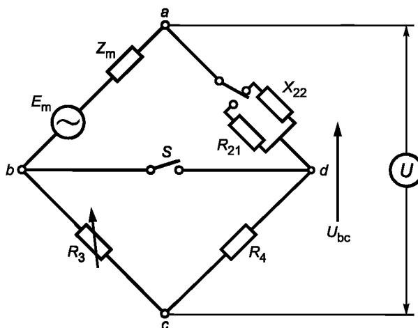
Рисунок Г.1 — Мостовая схема
