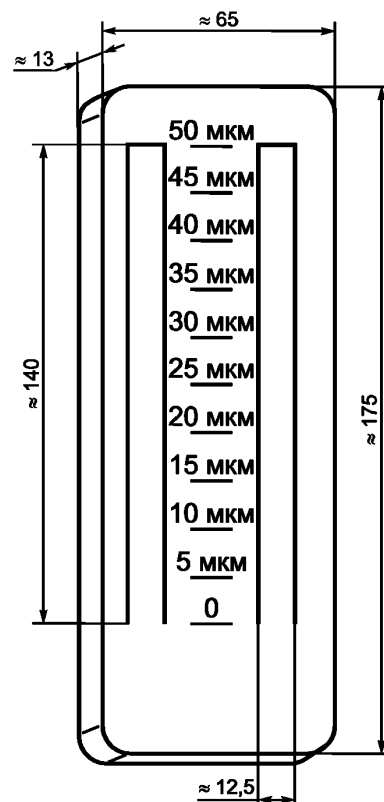
Рисунок 1 — Типовой прибор (гриндометр)
