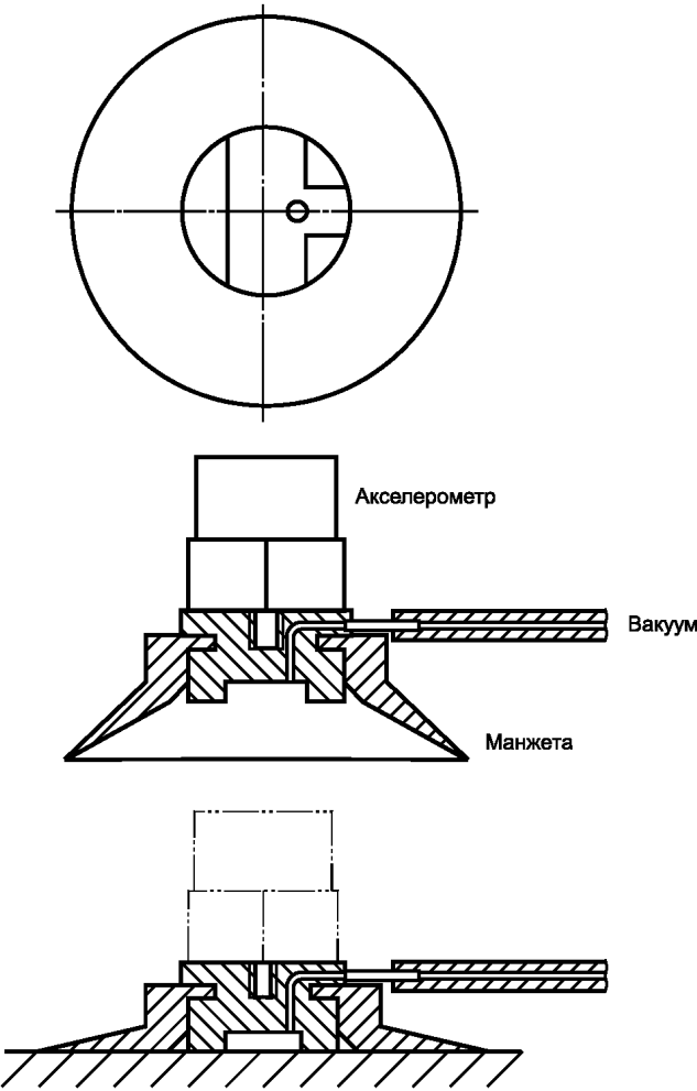
Рисунок 11— Вакуумное крепление
