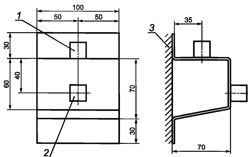
1 — образец для поверхности или полувстроенного крепления; 2 — образец полувстроенного крепления; 3 — монтажное приспособление
