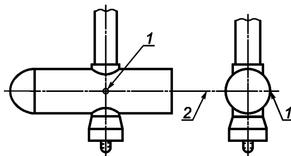
1 — измерительная точка; 2 — ось ударника
