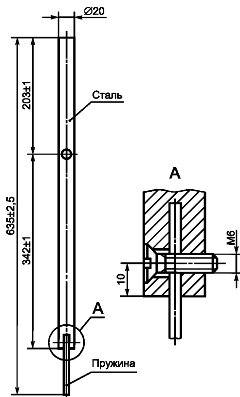
Рисунок Б.2 — Маятник
