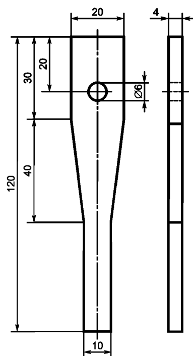
Рисунок Б.3 — Стальная пружина маятника
