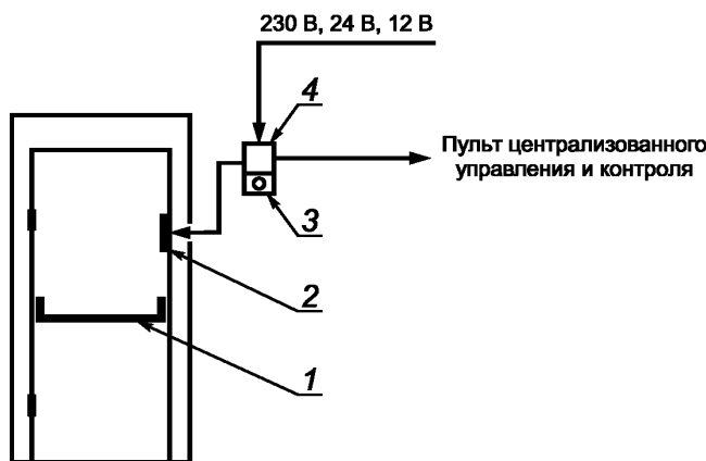
1 — основное замковое устройство «Антипаника», удерживающее дверь в закрытом состоянии; 2 — дополнительный электро-механический блокирующий механизм, разблокируется только электрическим сигналом; 3 — кнопка экстренного отпирания элемента 2; 4 — блок управления и контроля
