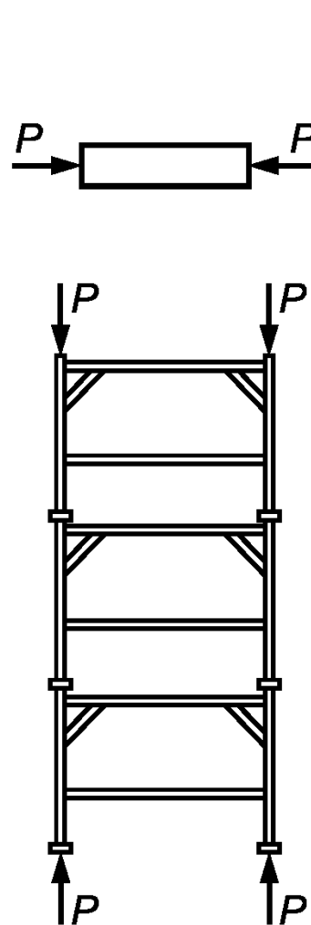
Рисунок 12 — Схемы испытания рам
