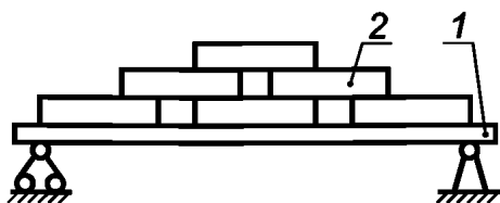
1 — испытательный образец; 2 — штучные грузы
