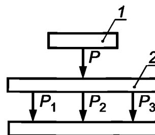
Рисунок 6 — Схема передачи нагрузок с помощью траверсы
