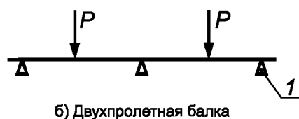
Рисунок 1 — Схемы приложения сосредоточенных нагрузок
