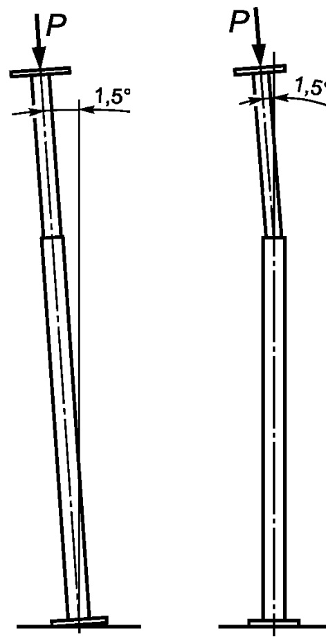
Рисунок 14 — Схема испытания составных стоек
