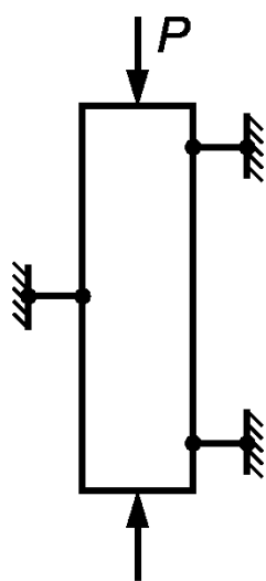
Рисунок 13 — Схемы закрепления стоек при испытании
