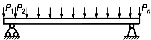
Рисунок 8 — Схема загрузки множеством P_1, P_2, \dots, P_n сосредоточенных нагрузок
