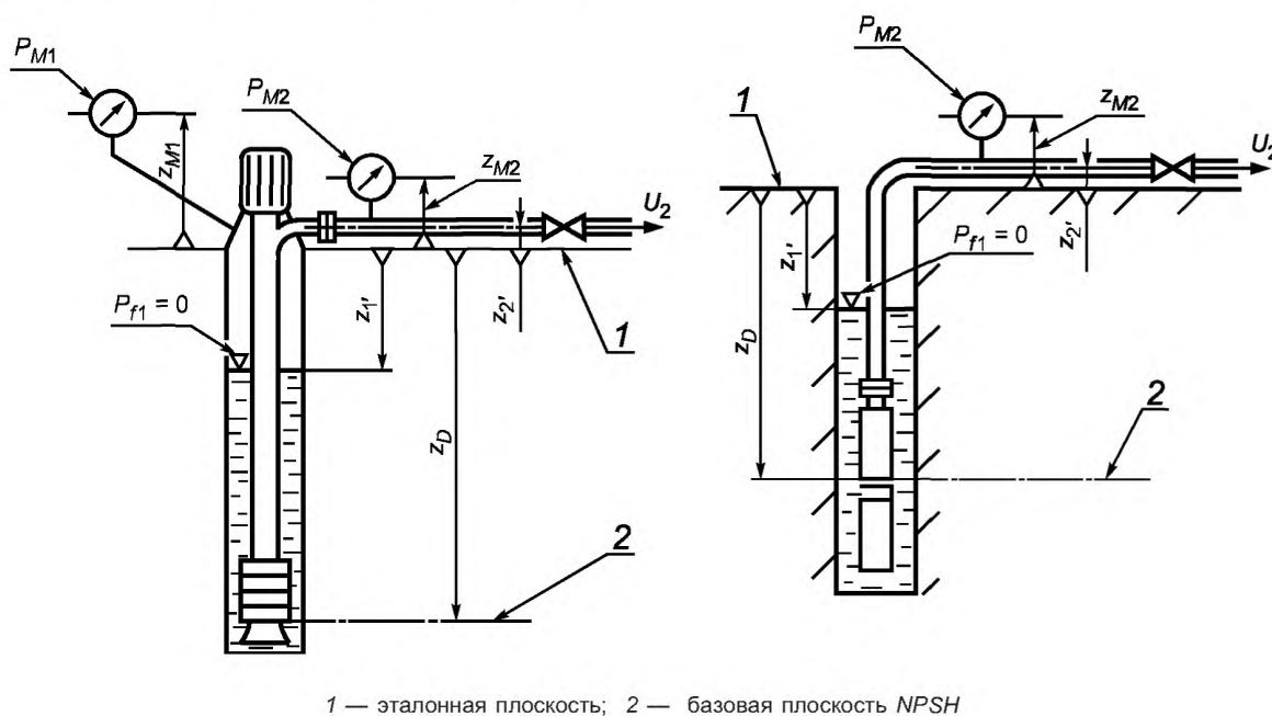
1 — эталонная плоскость; 2 — базовая плоскость NPSH
