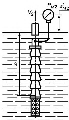
Рисунок 13.2
