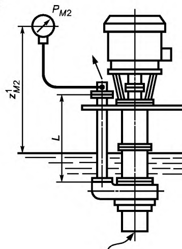
Рисунок 13.4
