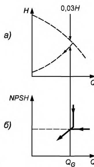
Рисунок 11.3
