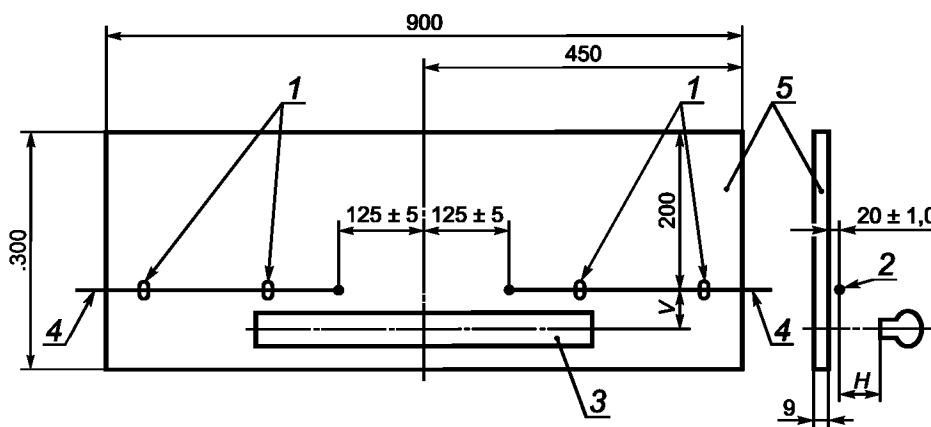
1 — опоры для термопар; 2 — кончик термопары; 3 — горелка; 4 — термопара типа К диаметром 1,5 мм в оболочке; 5 — испытательная стенка; H — расстояние кончика термопары от фронтальной поверхности горелки по горизонтали; V — расстояние кончика термопары от осевой линии горелки по вертикали
