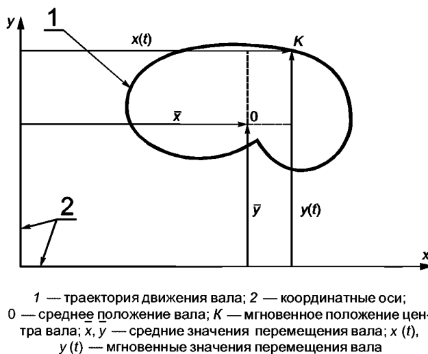
Рисунок 3 — Траектория движения вала
