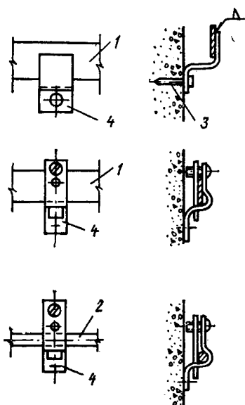
Рис. 7. Опоры для крепления заземляющих проводников
