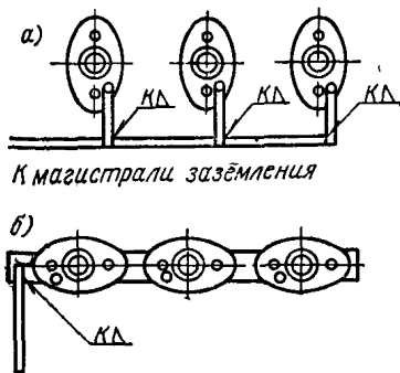
Рис. 19. Заземление опорных изоляторов
