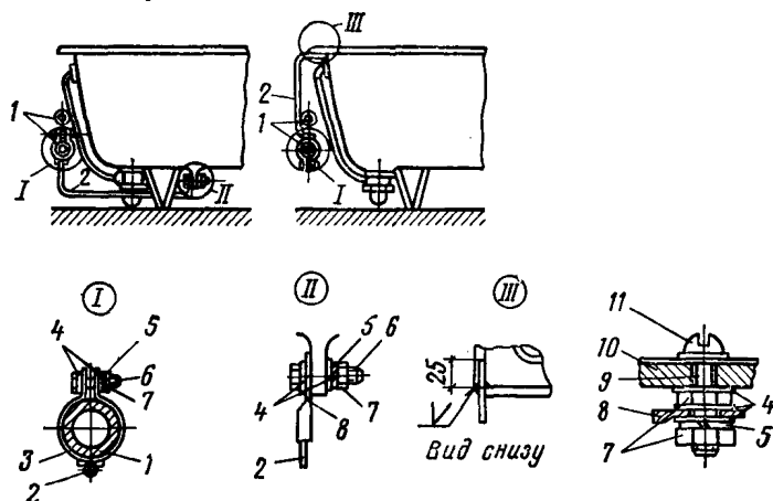
Рис. 29. Соединение металлического корпуса ванн с трубами водопровода
