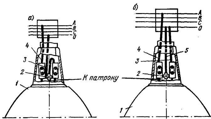
Рис. 23. Зануление корпусов светильников при глухозаземленной нейтрал
