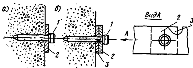
Рис. 6. Крепление заземляющих проводников из полосовой стали дюбелями с помощью строительного монтажного пистолета, пиротехнической или ручной оправки
