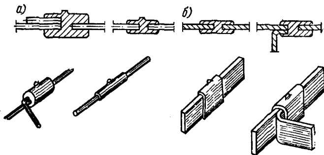
Рис. 11. Соединения заземляющих проводников, выполненные термитной сваркой
