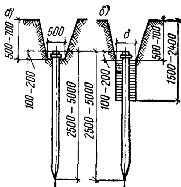
Рис. 15. Установка вертикальных заземлителей
