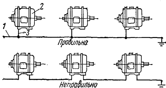
Рис. 1. Присоединение частей электроустановки к сети заземления (зануления)
