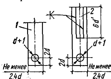
Рис. 21. Присоединение стальных заземляющих проводников к корпусам аппаратов
