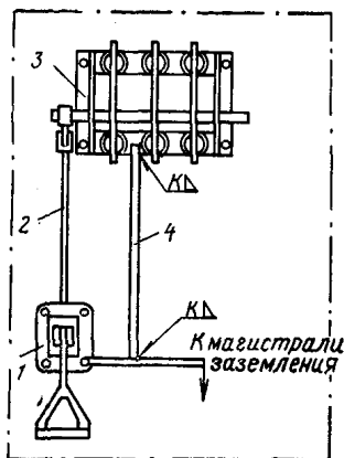
Рис. 20. Заземление рамы и привода трехполюсного разъединителя
