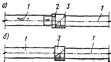
Рис. 3. Использование стальных труб в качестве заземляющих проводников
