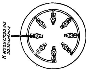
Рис. 16. Заземление опорных изоляторов нижней фазы бетонного реактора
