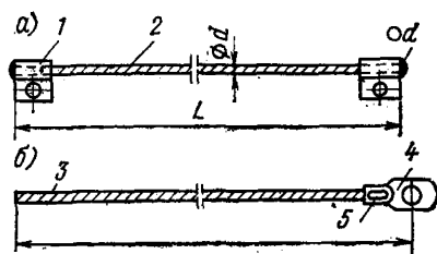
Рис. 2. Заземляющие перемычки
