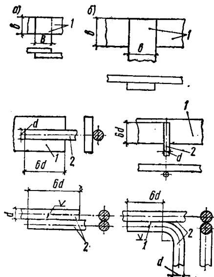
Рис. 5. Сварные соединения заземляющих проводников
