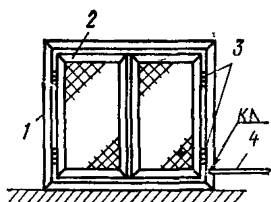
Рис. 18. Заземление рамы дверей
