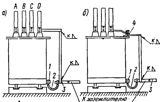
Рис. 17. Заземление силового трансформатора
