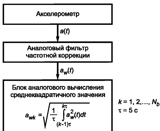
Рисунок 2 — Аналоговый метод расчета среднеквадратичного значения скорректированного ускорения
