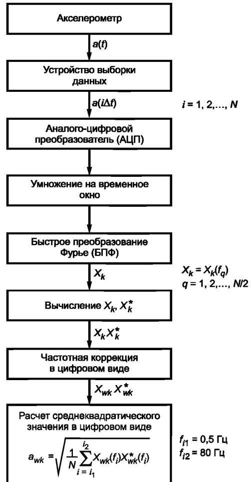
Рисунок 4 — Цифровой метод расчета среднеквадратического значения скорректированного ускорения
