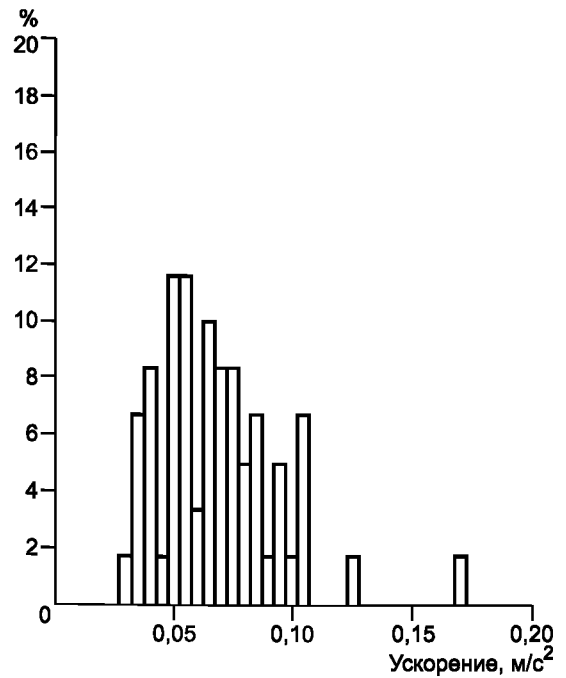
а) Подушка сиденья, направление X
