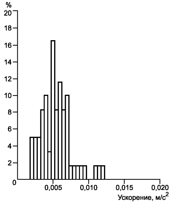
с) Подушка сиденья, направление Z
