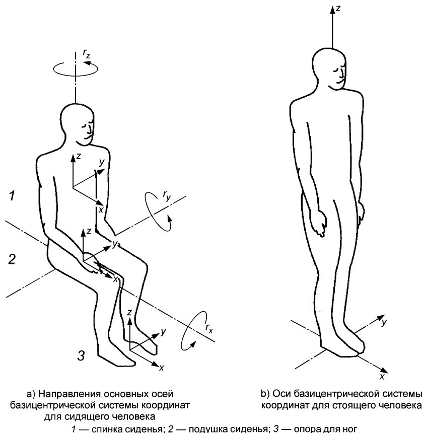
Рисунок 1 — Базицентральная система координат для тела человека
