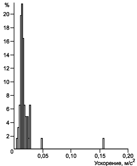
d) Спинка сиденья, направление X
